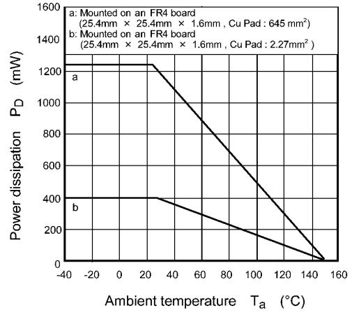
Fig. 9.14 P_D - T_a
