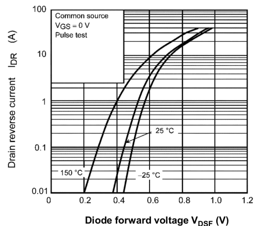
Fig. 9.12 I_{DR} - V_{DSF}
