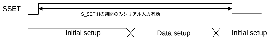
図 7.2 SSET 入力タイミングチャート
