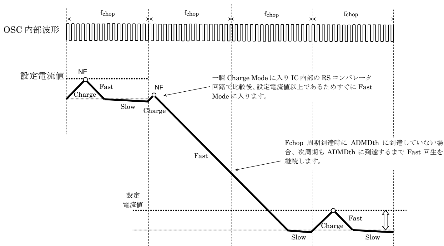
図 5.9 ADMD 電流波形 (1 周期到達する場合)
