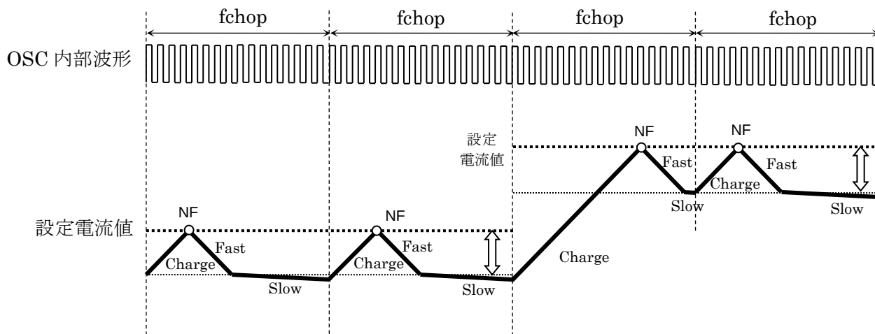
図 5.6 ADMD 電流波形
