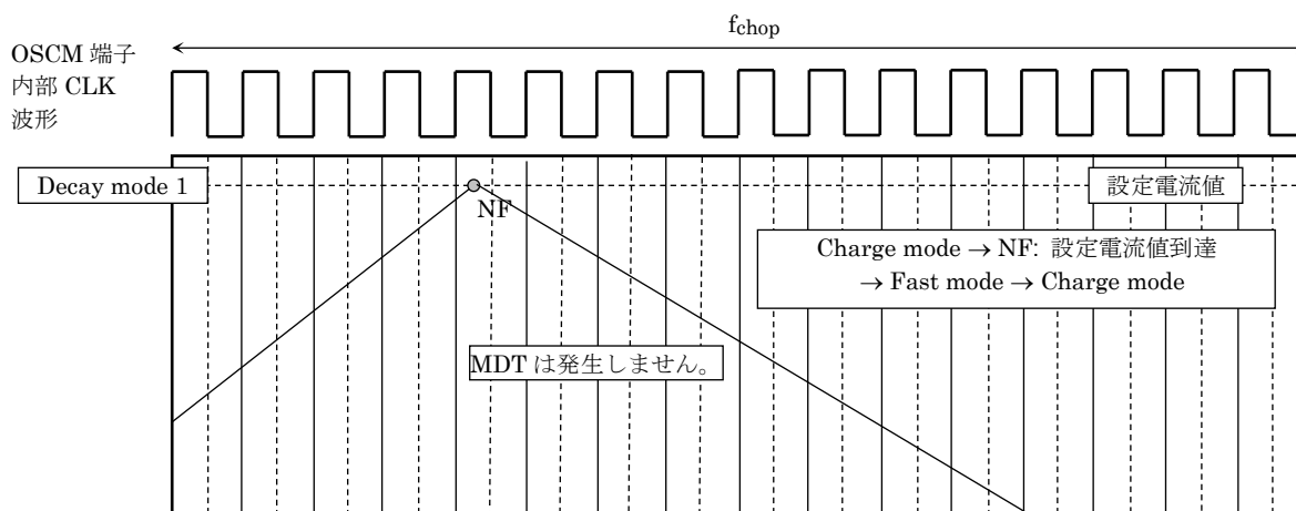
図 5.2 Fast decay 制御
