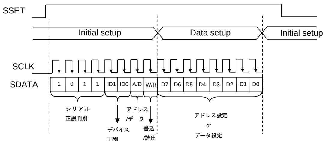
図 7.1 シリアル入力タイミングチャート
