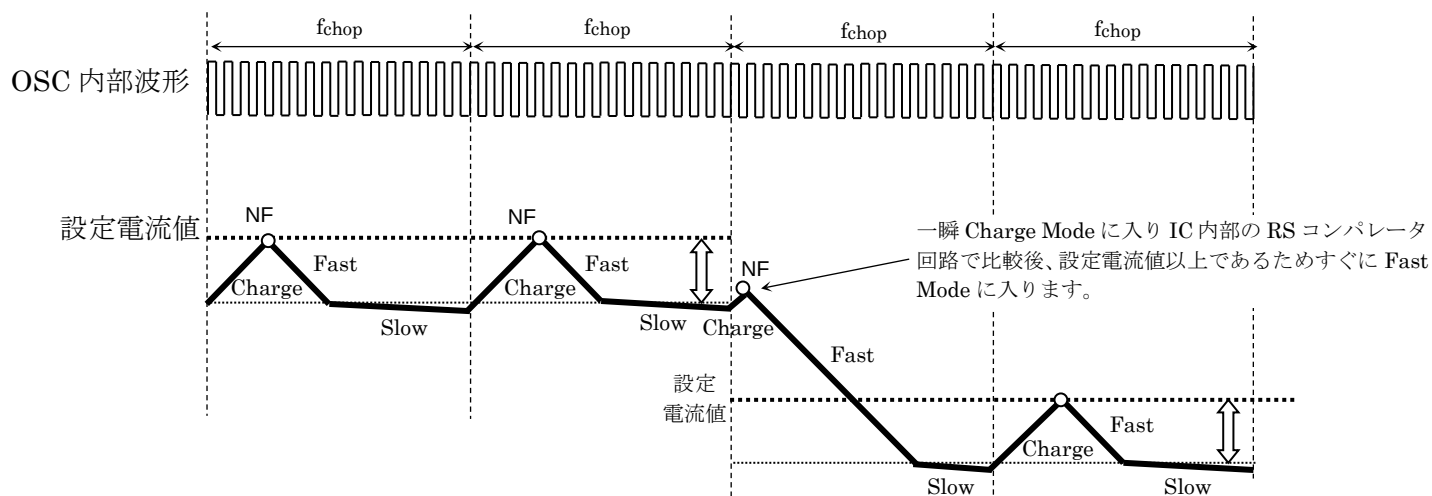
図 5.8 ADMD 電流波形 (設定電流値が減少方向の場合)
