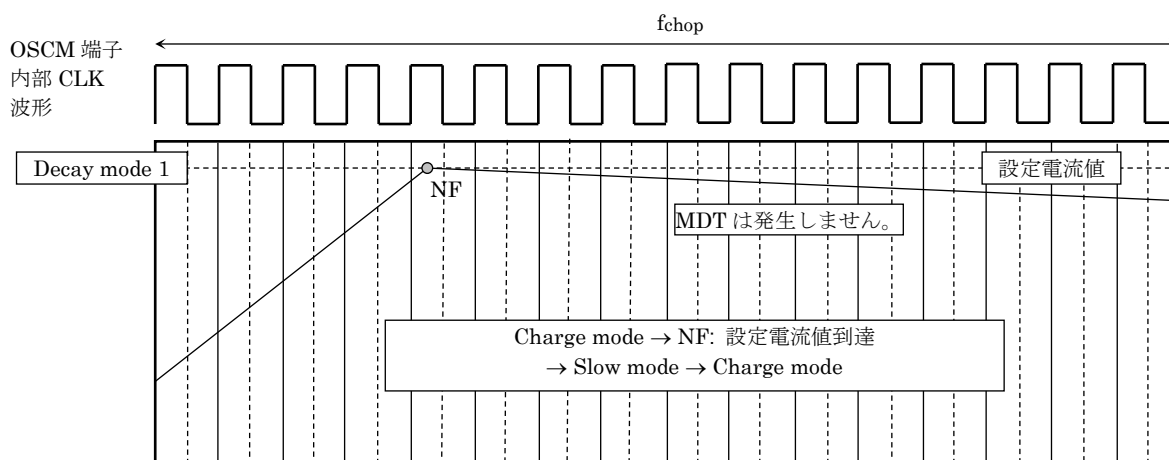
図 5.3 Slow decay 制御
