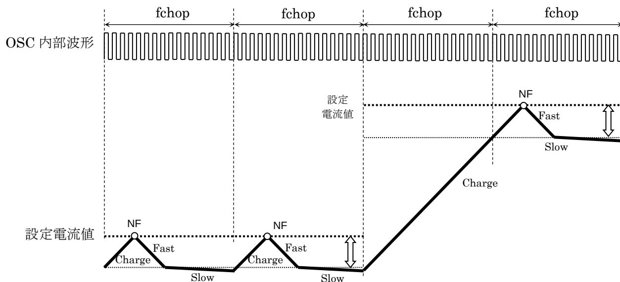
図 5.7 ADMD 電流波形 ( f_{chop} 1 周期以上の場合)
