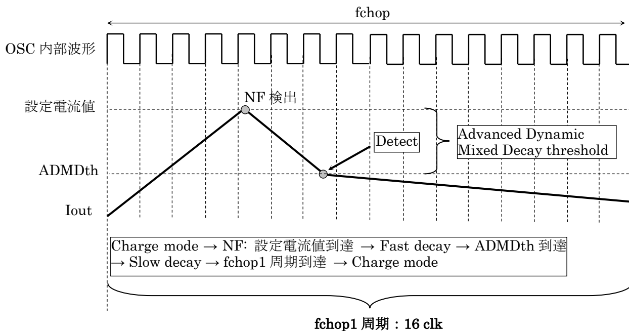
図 5.4 ADMD 制御
