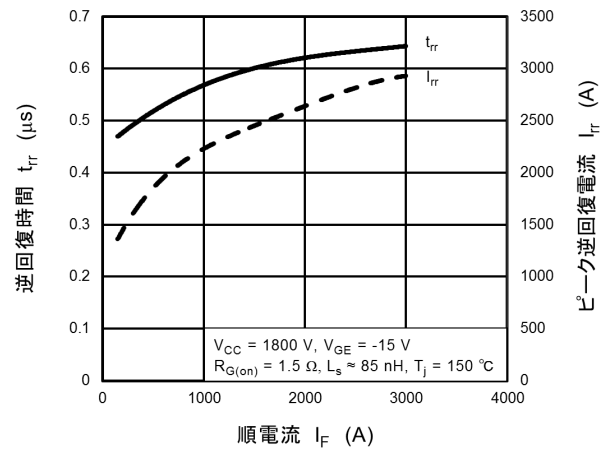
図 7.10 t_{rr}, I_{rr} - I_F
