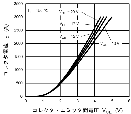
図 7.2 出力特性
