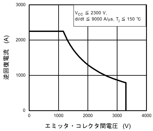
図 7.16 RRSOA(最大値(保証値))
