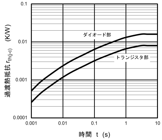
図 7.14 r_{th(j-c)} - t (最大値(保証値))
