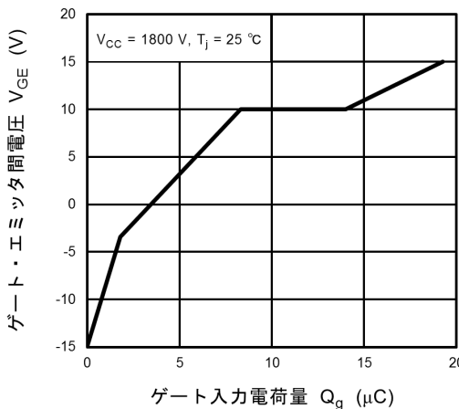
図 7.5 V_{GE} - Q_g
