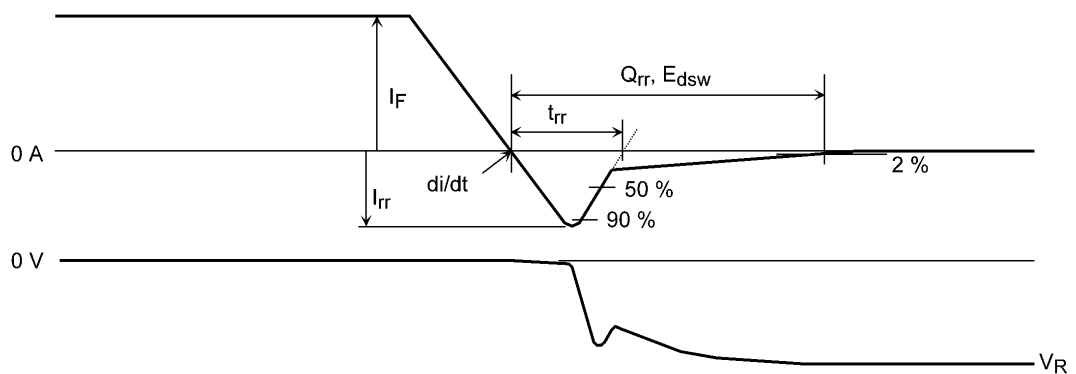
図 6.3 タイミングチャート(ダイオード部)
