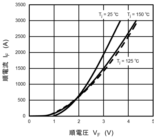
図 7.3 I_f - V_f
