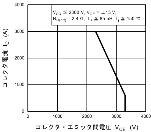
図 7.15 RBSOA(最大値(保証値))
