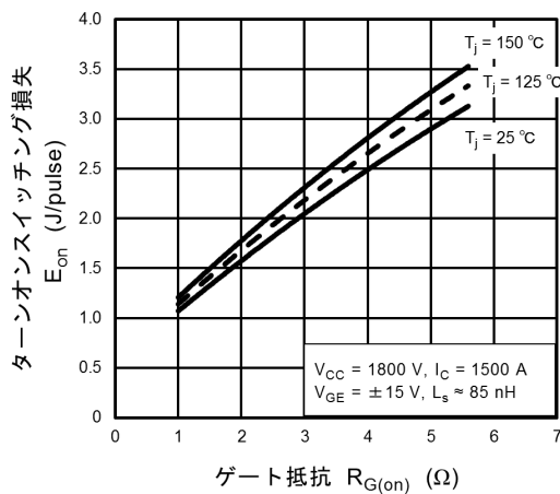
図 7.11 E_{on} - R_{G(on)}
