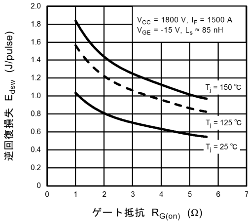
図 7.13 E_{dsw} - R_{G(on)}
