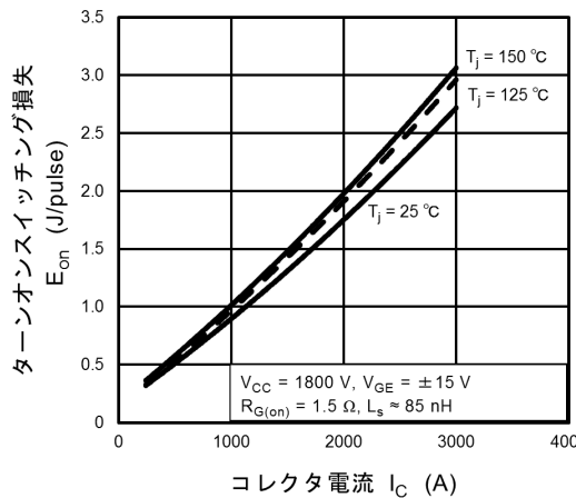
図 7.6 E_{on} - I_c
