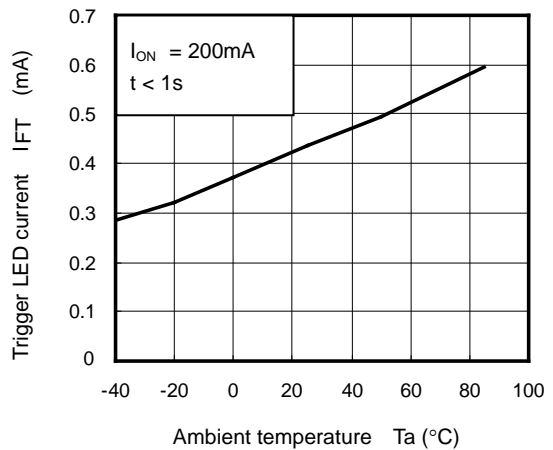
I_{FT} - T_a
