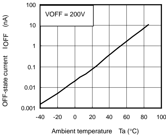
I_{OFF} - T_a
