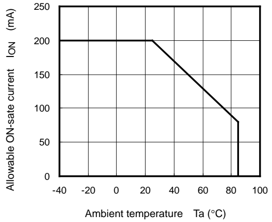
I_{ON} - T_a
