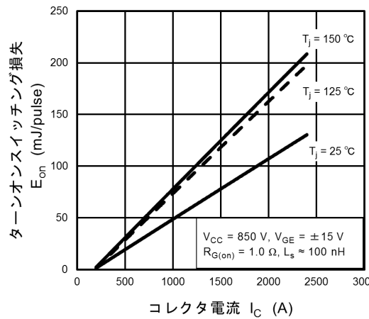
図 7.6 E_{on} - I_C
