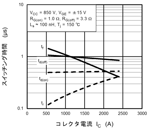
図 7.9 t_{d(on)}, t_r, t_{d(off)}, t_f - I_C
