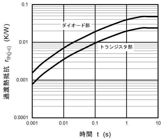
図 7.13 r_{th(j-c)} - t (最大値(保証値))
