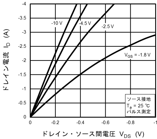
図 7.1 I_D - V_{DS}
