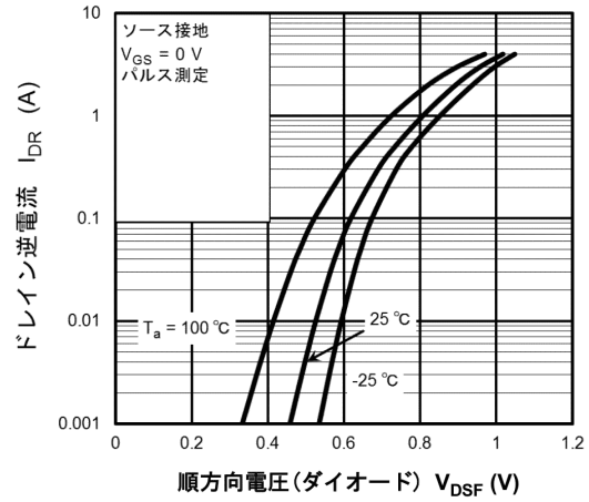
図 7.8 I_{DR} - V_{DSF}
