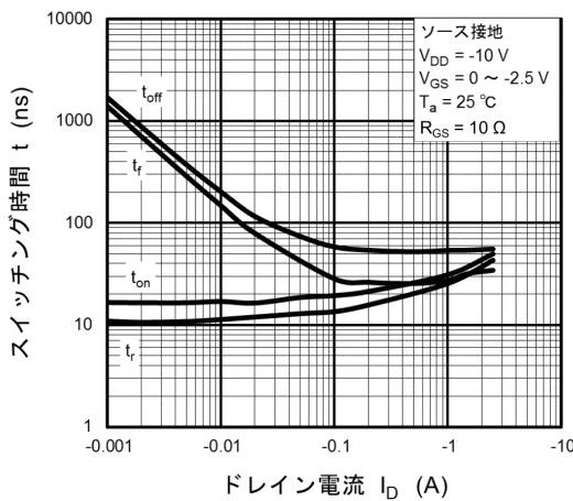
図 7.11 t - I_D
