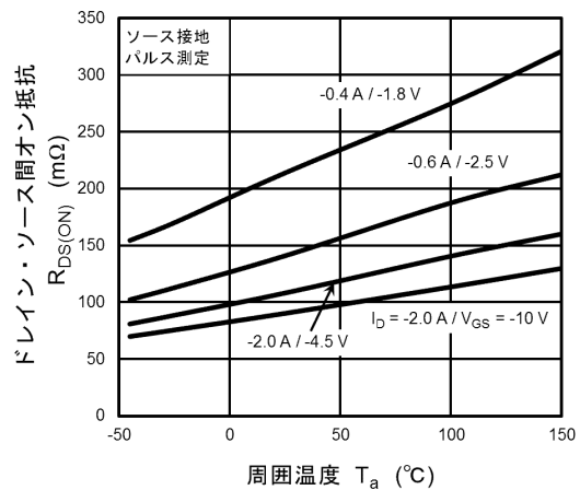
図 7.6 R_{DS(ON)} - T_a
