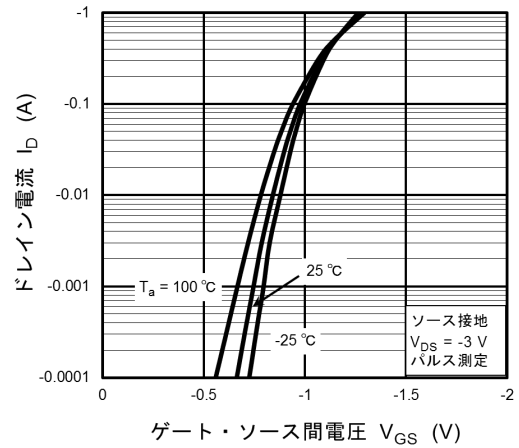
図 7.2 I_D - V_{GS}
