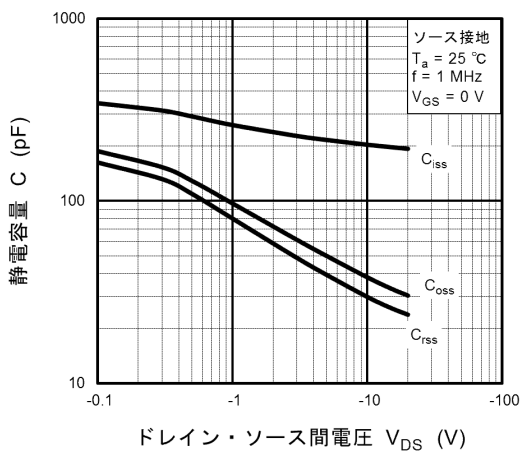
図 7.9 C - V_{DS}
