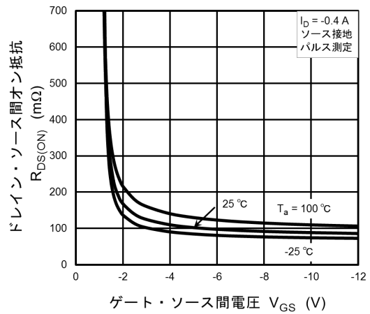
図 7.4 R_{DS(ON)} - V_{GS}
