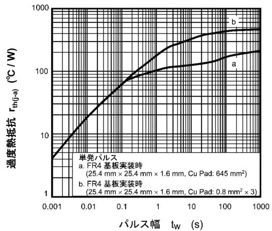
図 7.12 r_{th(j-a)} - t_w
