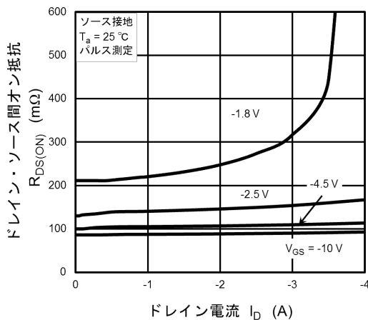
図 7.5 R_{DS(ON)} - I_D
