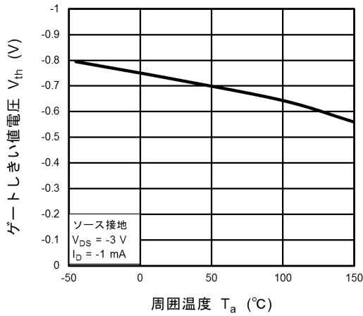
図 7.7 V_{th} - T_a
