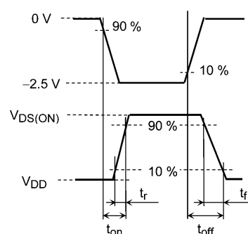
図 5.3.2 入力波形/出力波形
