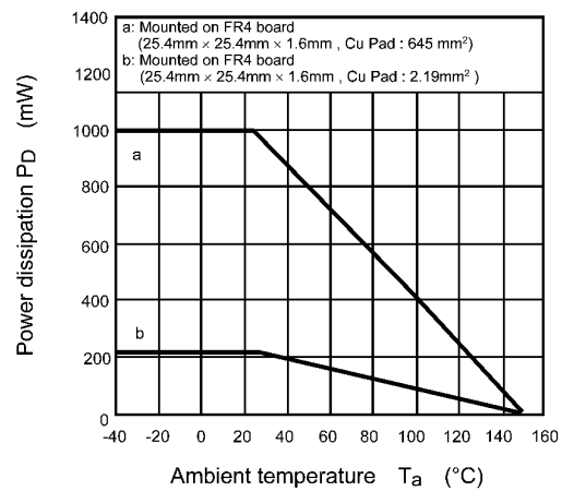
Fig. 9.12 P_D - T_a
