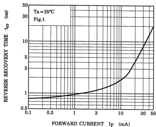
Fig. 7.4 t_{rr} - I_F
