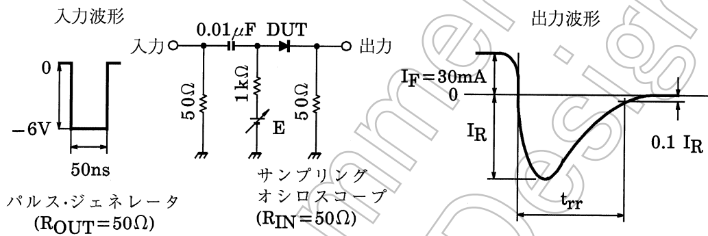
図 1. 逆回復時間 (t rr ) 測定回路
