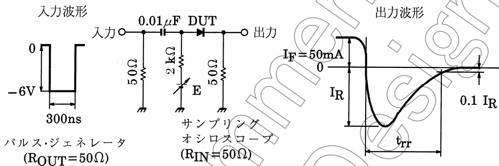
図 1. 逆回復時間 (t rr ) 測定回路
