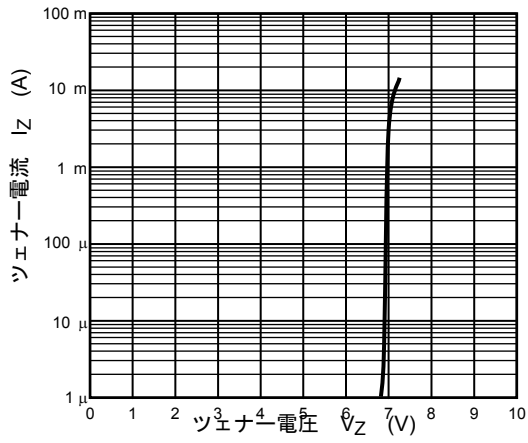
I_Z - V_Z
