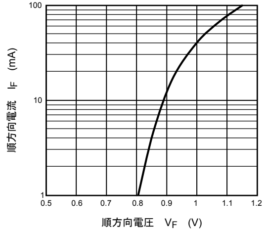
I_F - V_F
