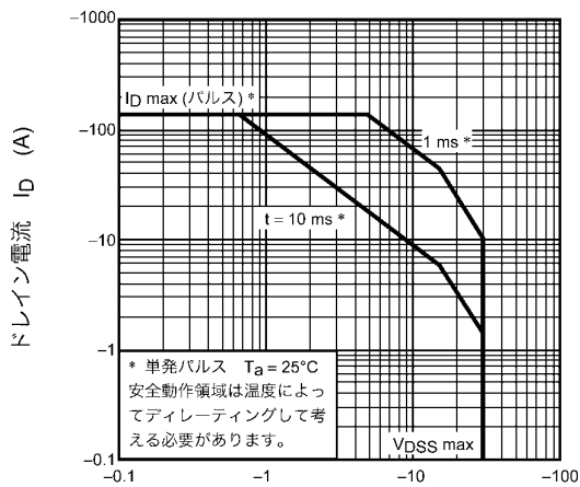
ドレイン・ソース間電圧 V_{DS} (V) 図 8.14 安全動作領域 (最大値 (保証値))
