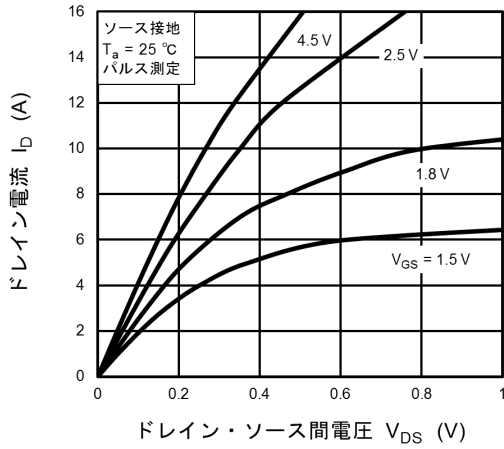
図 9.1.1 I_D - V_{DS}
