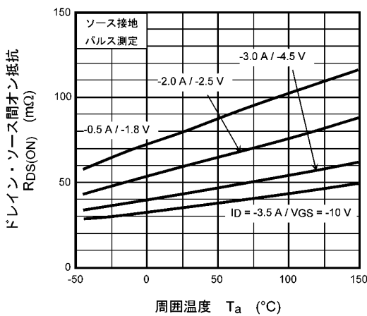
図 9.2.5 R_{DS(ON)} - T_a
