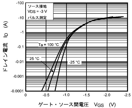
図 9.2.2 I_D - V_{GS}
