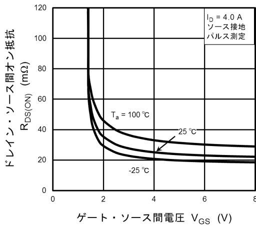
図 9.1.3 R_{DS(ON)} - V_{GS}
