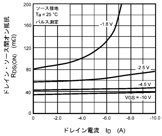
図 9.2.4 R_{DS(ON)} - I_D
