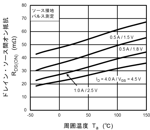
図 9.1.5 R_{DS(ON)} - T_a
