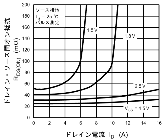
図 9.1.4 R_{DS(ON)} - I_D
