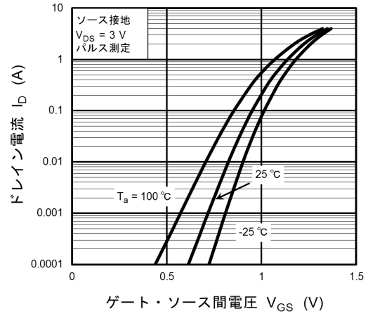
図 9.1.2 I_D - V_{GS}
