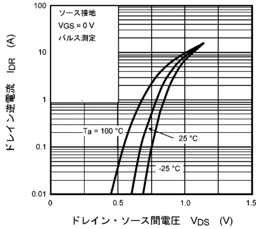
図 9.2.7 I_{DR} - V_{DS}
