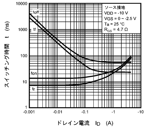
図 9.2.8 t - I_D
