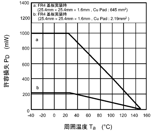
図 9.3.2 P_D - T_a
