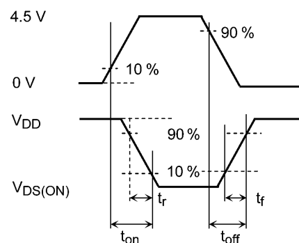
入力波形/出力波形
