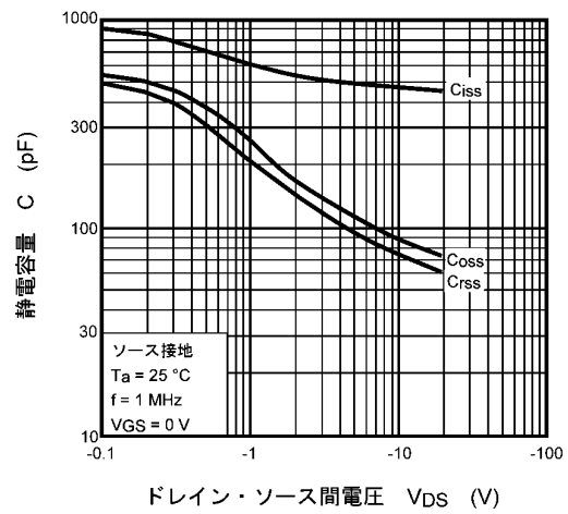
図 9.2.10 C - V_{DS}
