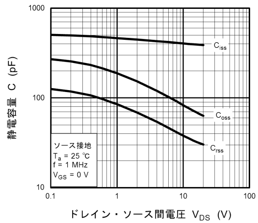
図 9.1.10 C - V_{DS}
