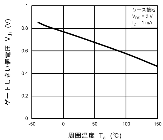
図 9.1.6 V_{th} - T_a
