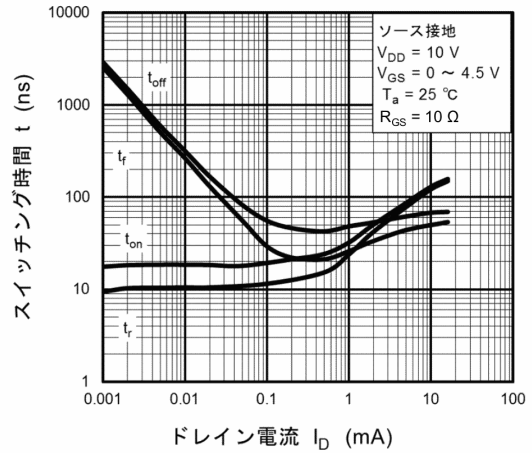
図 9.1.8 t - I_D
