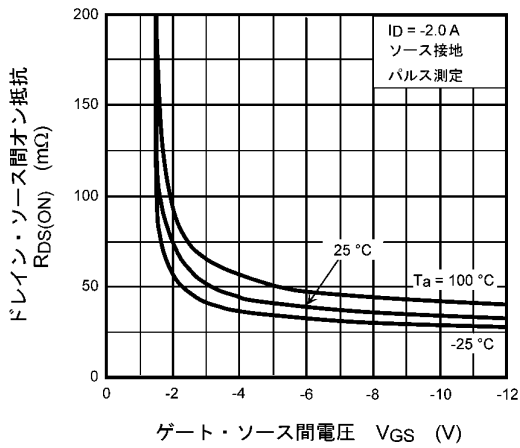
図 9.2.3 R_{DS(ON)} - V_{GS}
