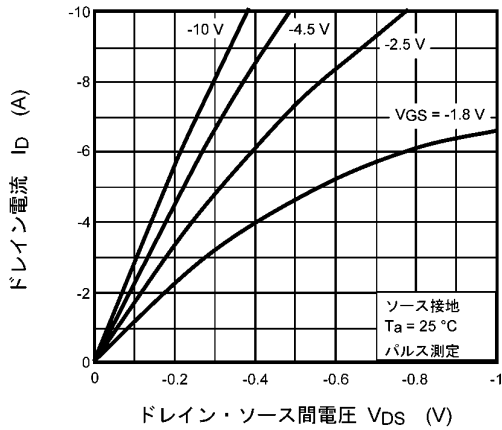
図 9.2.1 I_D - V_{DS}
