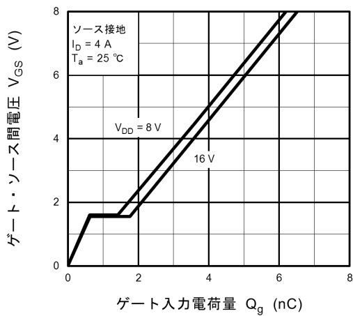
図 9.1.9 ダイナミック入力特性
