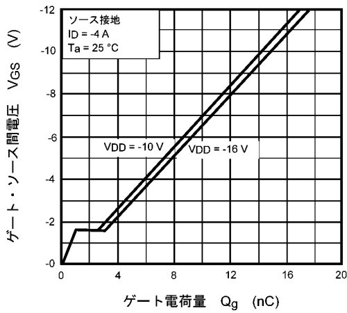
図 9.2.9 ダイナミック入力特性
