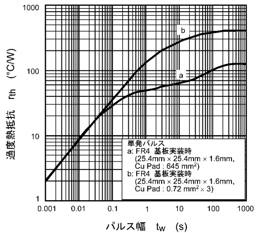
図 7.12 r_{th} - t_w
