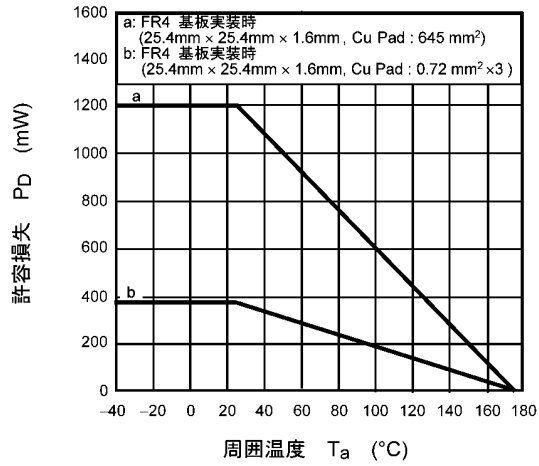
図 7.13 P_D - T_a
