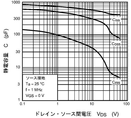
図 7.8 C - V_{DS}
