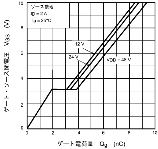
図 9.10 ダイナミック入力特性
