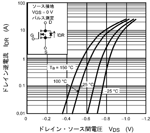
図 7.7 I_{DR} - V_{DS}
