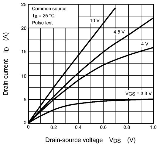
Fig. 9.1 I_D - V_{DS}
