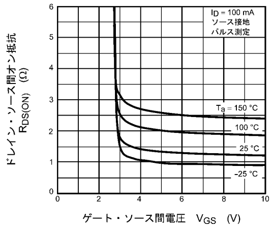
図 8.4 R_{DS(ON)} - V_{GS}
