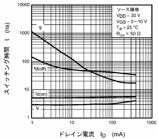
図 8.10 t - I_D
