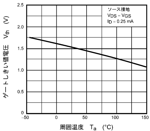
図 8.6 V_{th} - T_a
