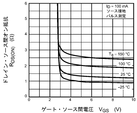
図 7.4 R_{DS(ON)} - V_{GS}
