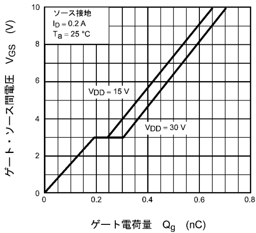
図 8.9 ダイナミック入力特性
