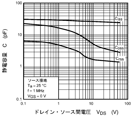
図 7.7 C - V_{DS}
