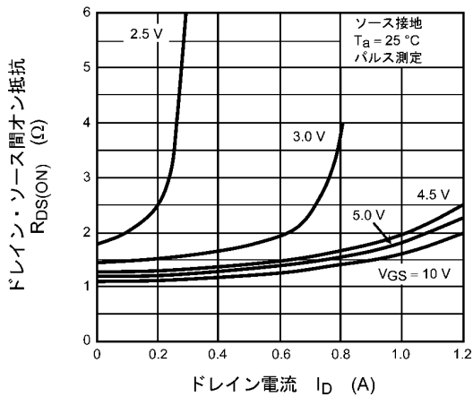
図 7.3 R_{DS(ON)} - I_D
