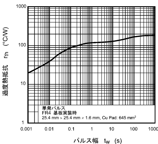
図 8.11 r_{th} - t_w
