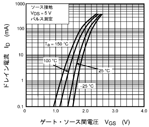
図 7.2 I_D - V_{GS}
