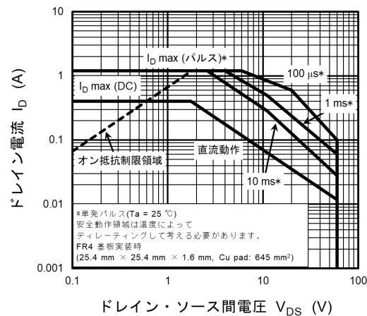
図 8.12 安全動作領域
