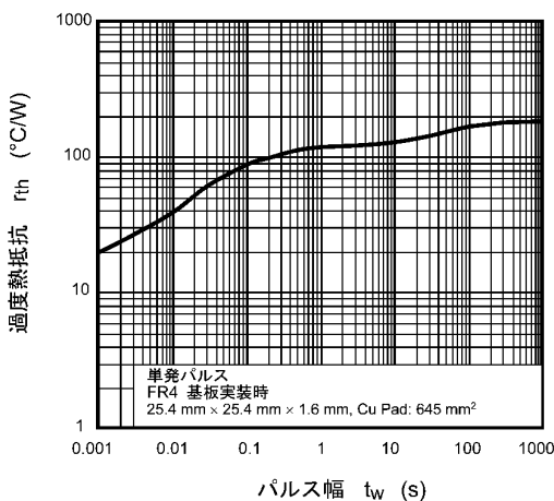
図 7.11 r_{th} - t_w
