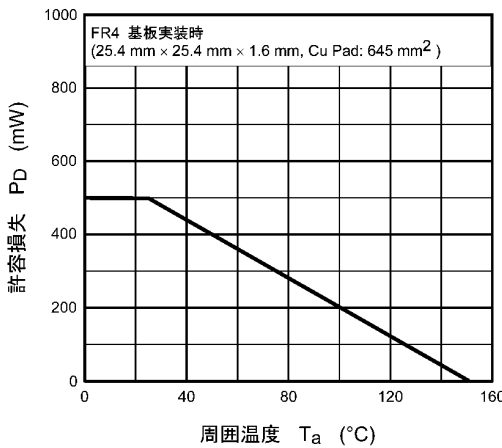
図 8.11 P_D - T_a
