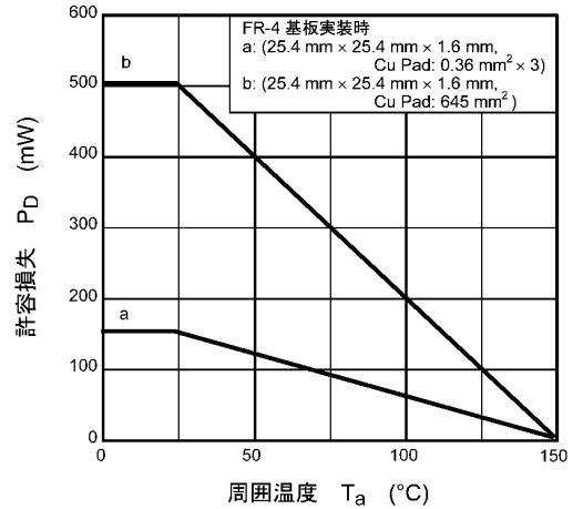
図 8.12 P_D - T_a
