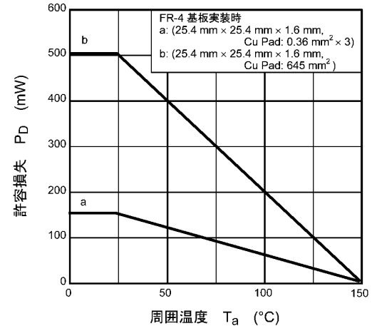
図 7.12 P_D - T_a
