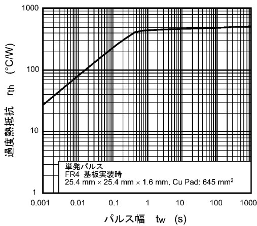
図 7.11 r_{th} - t_w
