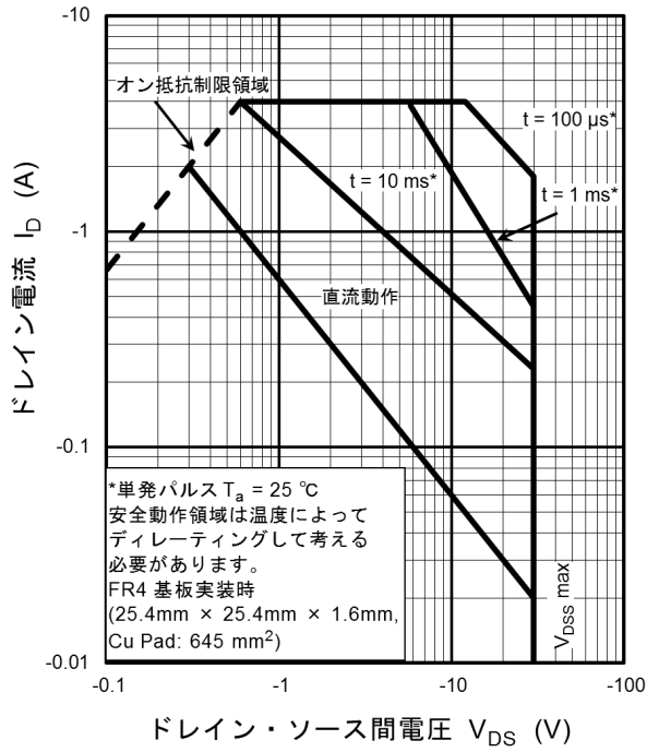
図 7.13 安全動作領域
