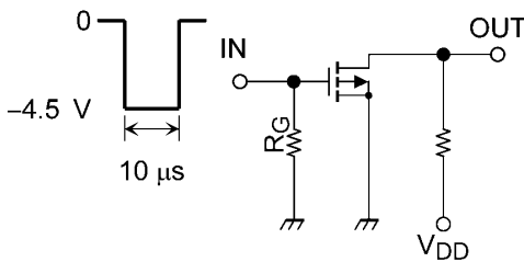
図 5.3.1 スwitching時間の測定回路
