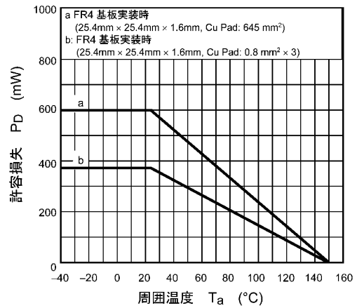
図 7.12 P_D - T_a
