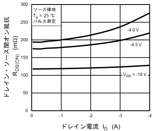
図 7.4 R_{DS(ON)} - I_D
