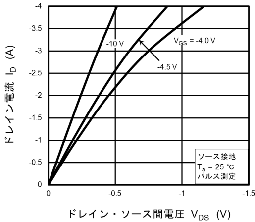
図 7.1 I_D - V_{DS}
