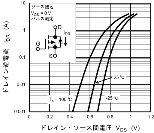
図 7.7 I_{DR} - V_{DS}
