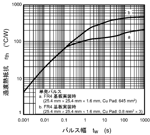
図 7.11 r_{th} - t_w
