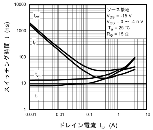
図 7.10 t - I_D
