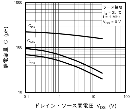
図 7.8 C - V_{DS}
