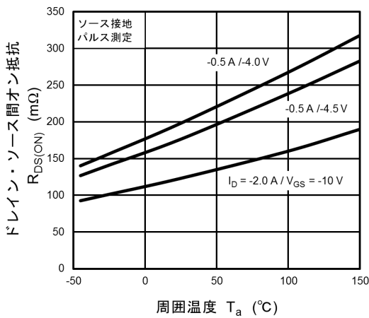
図 7.5 R_{DS(ON)} - T_a
