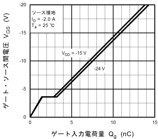
図 7.9 ダイナミック入力特性
