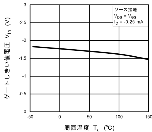
図 7.6 V_{th} - T_a
