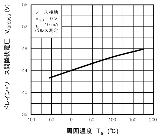
図 9.12 V_{(BR)DSS} - T_a
