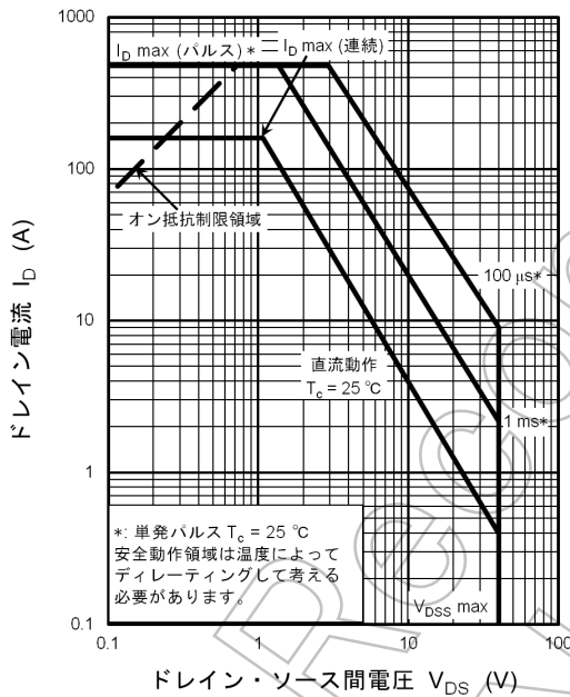
図 9.14 安全動作領域 (最大値 (保証値))
