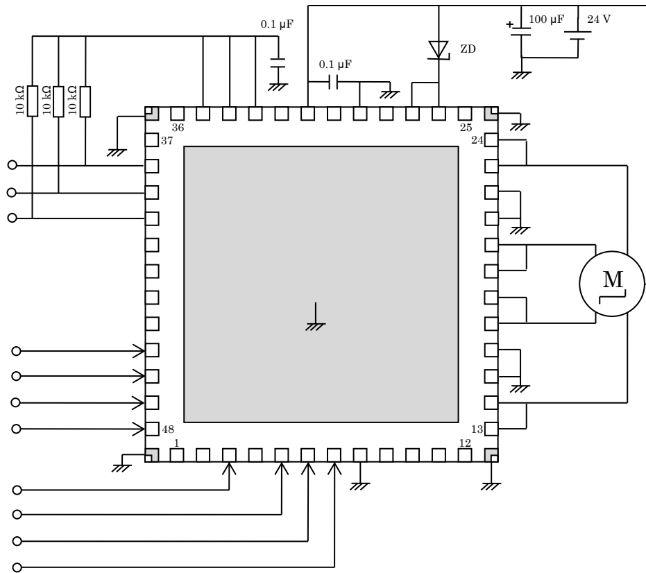
図 10.2 応用回路例 (定電圧制御)
