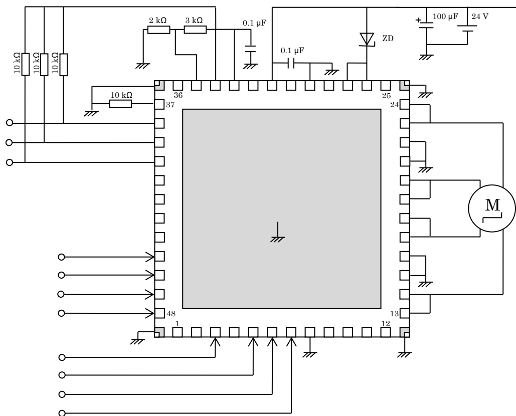
図 10.1 応用回路例 (定電流制御)
