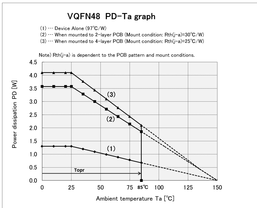
図 7 PD - Ta (パッケージの許容損失)
