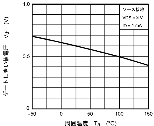
図 8.6 V_{th} - T_a
