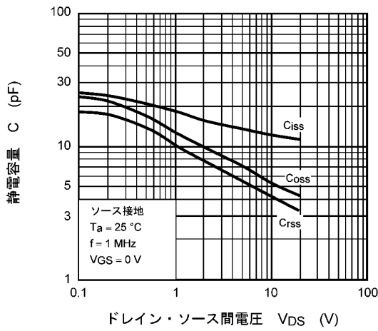
図 8.9 C - V_{DS}
