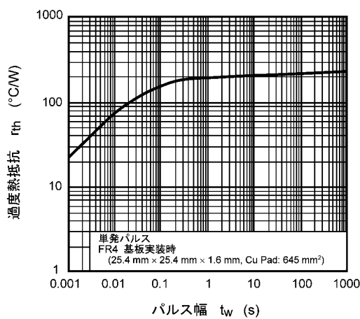
図 8.11 r_{th} - t_w
