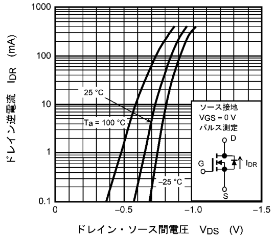
図 8.8 I_{DR} - V_{DS}
