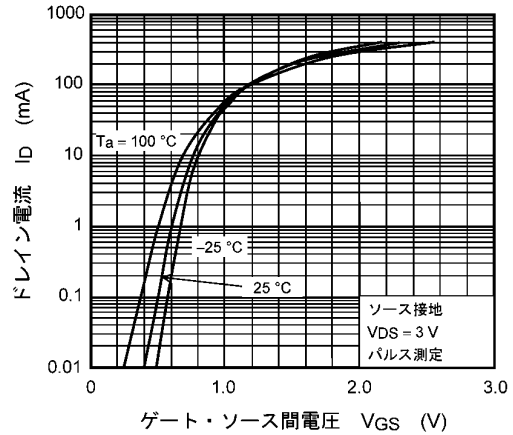
図 8.2 I_D - V_{GS}
