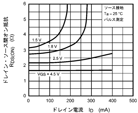
図 8.4 R_{DS(ON)} - I_D
