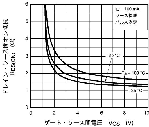
図 8.3 R_{DS(ON)} - V_{GS}
