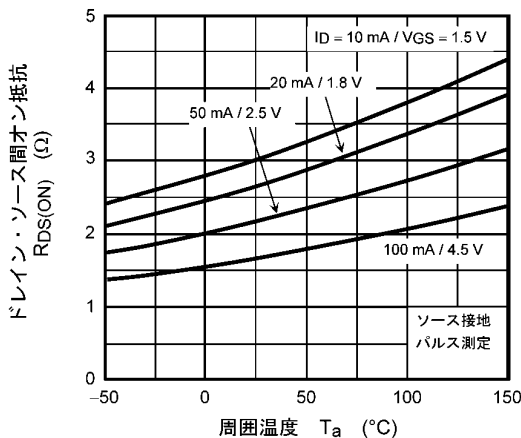
図 8.5 R_{DS(ON)} - T_a
