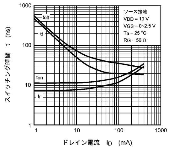
図 8.10 t - I_D
