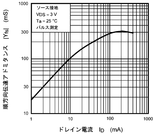
図 8.7 |Y_{fs}| - I_D
