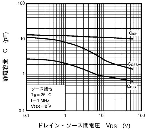
図 7.7 C - V DS
