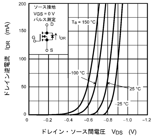
図 7.8 IDR - V DS
