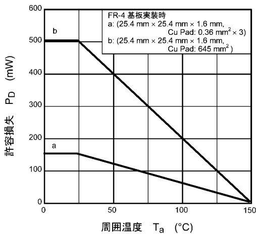
図 7.11 P D - T a
