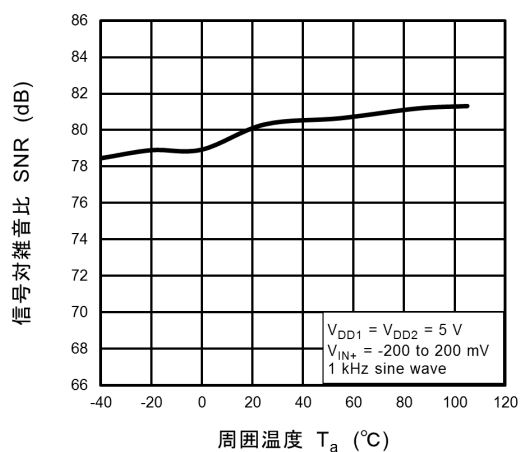
図 12.4 SNR - T_a
