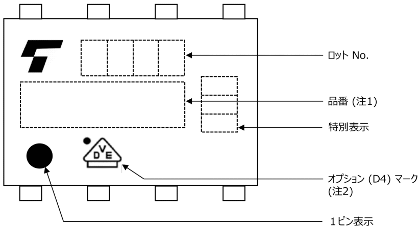
図 16.3 現品表示例
