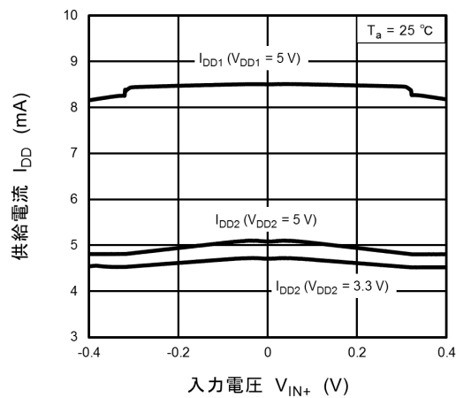
図 12.6 I_{DD} - V_{IN+}
