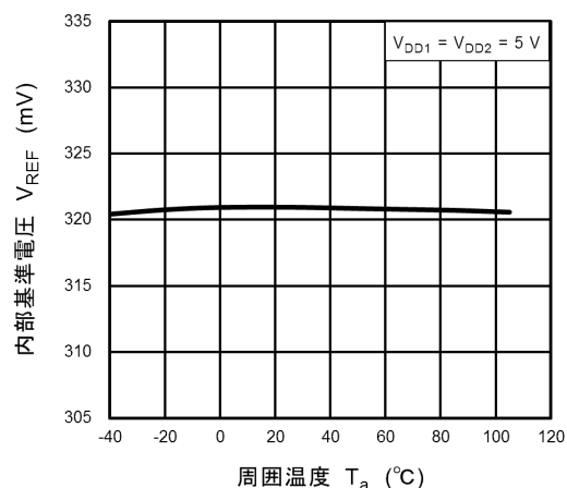
図 12.2 V_{REF} - T_a
