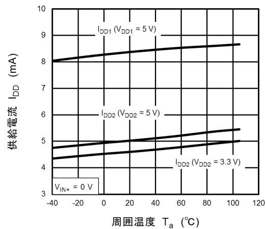
図 12.7 I_{DD} - T_a
