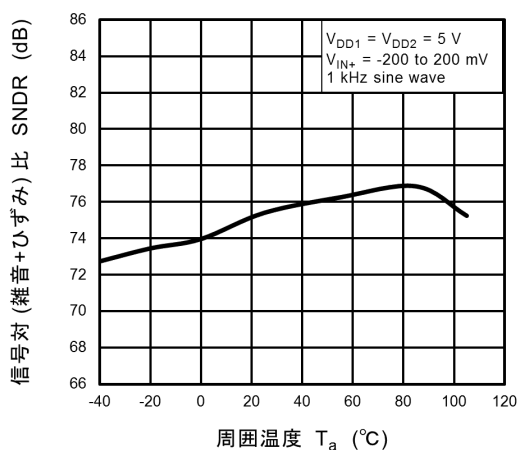
図 12.5 SNDR - T_a
