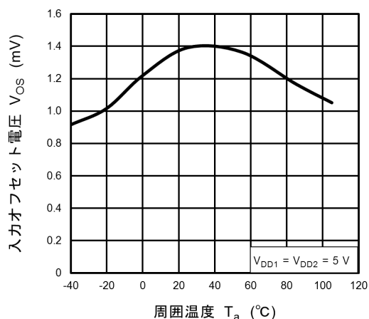
図 12.1 V_{OS} - T_a
