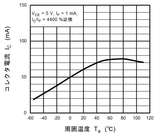
図 11.12 I_C - T_a
