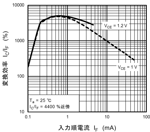
図 11.11 I_C/I_F - I_F
