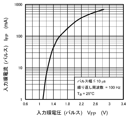
図 11.6 I_{FP} - V_{FP}
