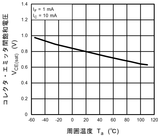
図 11.9 V_{CE(sat)} - T_a
