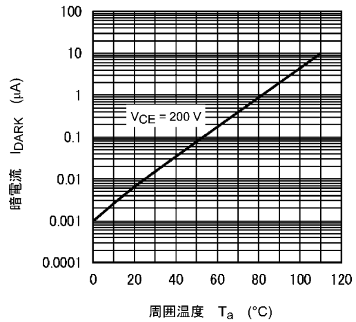
図 11.8 I_{DARK} - T_a
