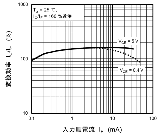
図 11.12 I_C/I_F - I_F
