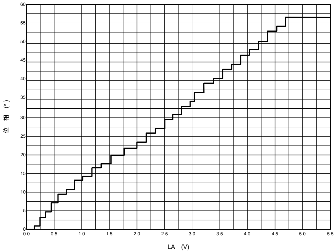
LA (V) - 進角 (°) 特性
