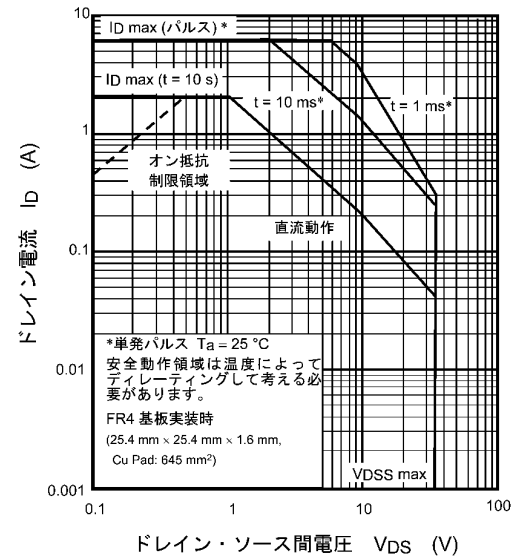
図 7.12 安全動作領域
