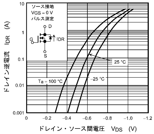
図 7.8 I_{DR} - V_{DS}
