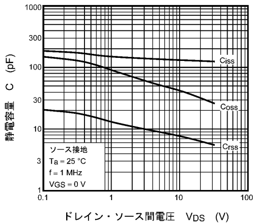
図 7.9 C - V_{DS}
