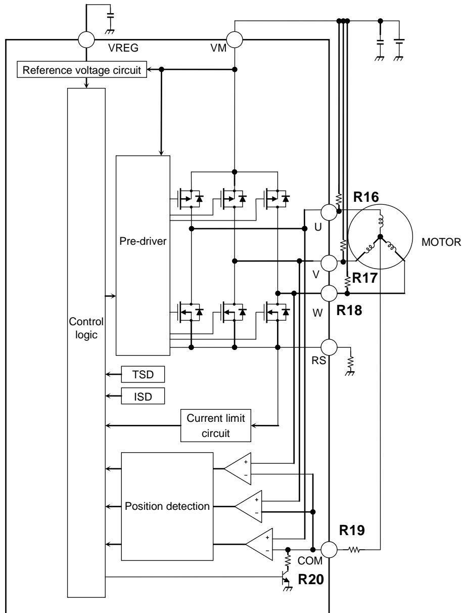
Figure 2 参考回路例
