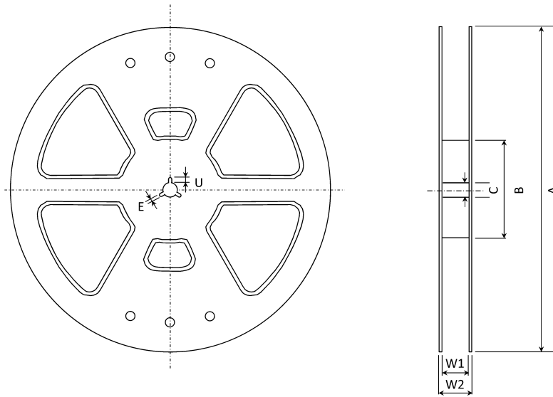
Fig. 16.3.5.1 Reel dimension
