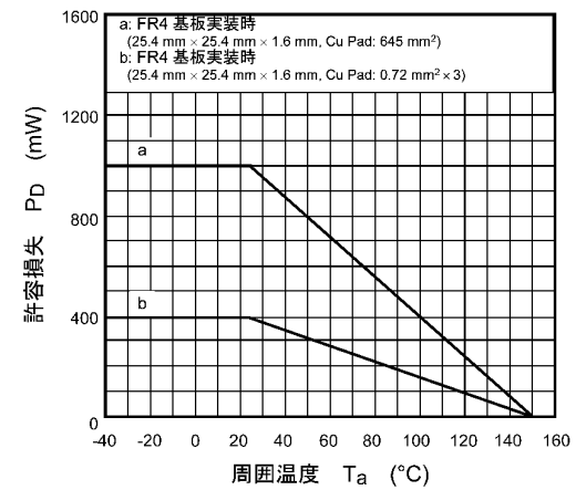
図 8.12 P_D - T_a
