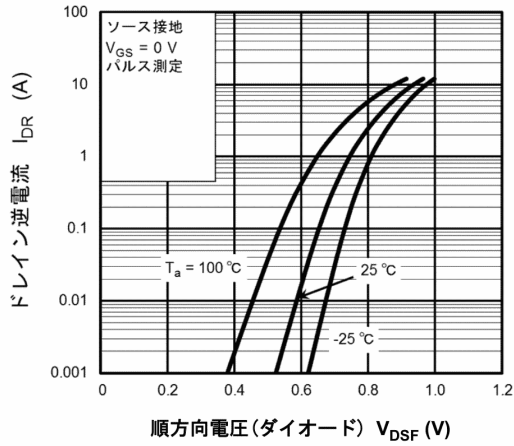
図 8.7 I_{DR} - V_{DSF}
