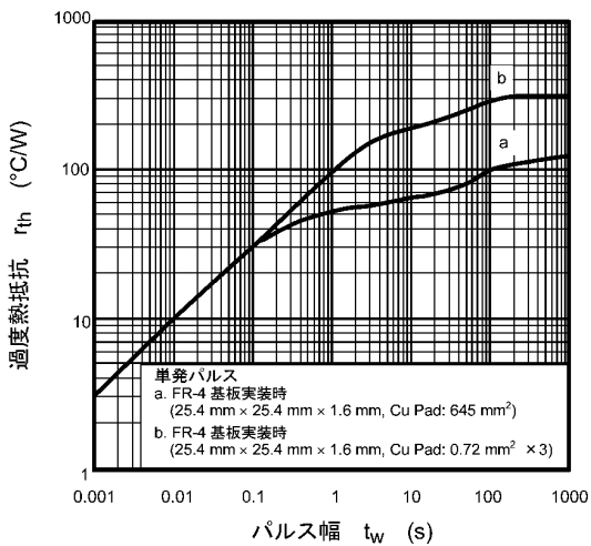
図 8.11 r_{th} - t_w
