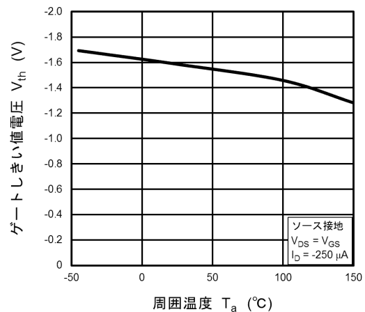
図 8.6 V_{th} - T_a
