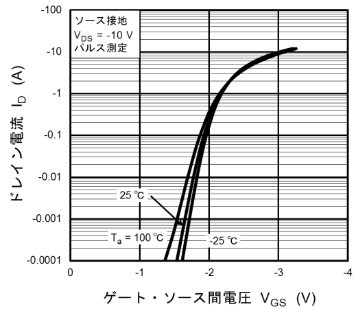
図 7.2 I_D - V_{GS}
