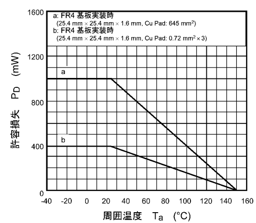
図 7.12 P_D - T_a
