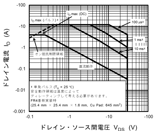
図 8.13 安全動作領域
