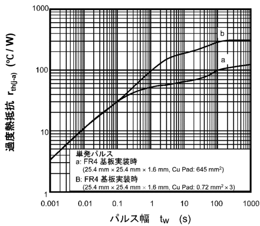
図 8.11 r_{th(j-a)} - t_w
