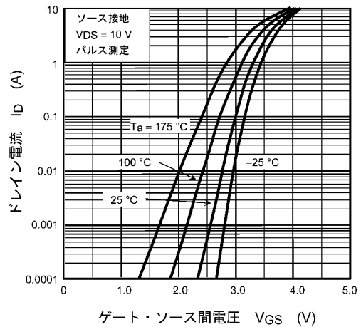
図 7.2 I_D - V_{GS}
