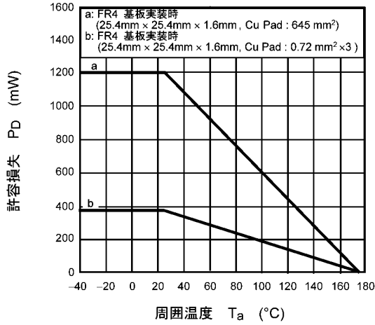
図 8.13 P_D - T_a
