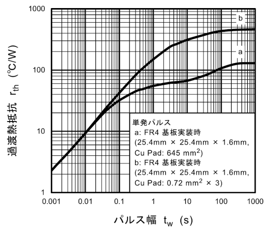
図 9.12 r_{th} - t_w
