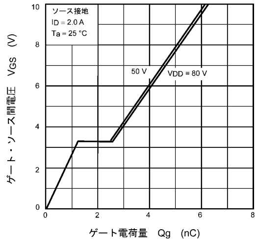
図 9.10 ダイナミック入力特性
