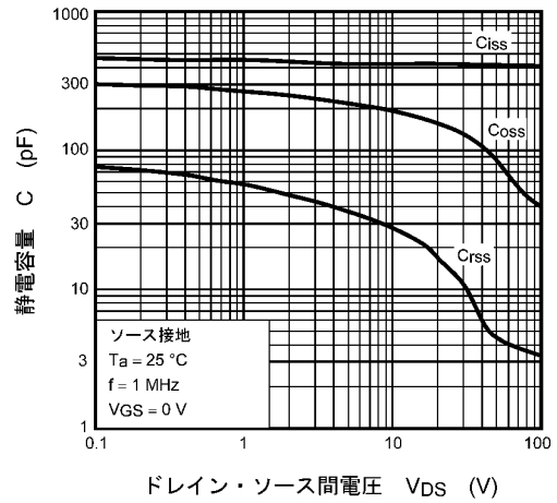
図 8.8 C - V_{DS}
