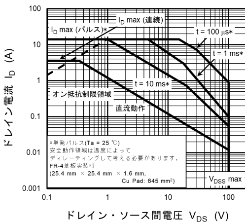
図 9.11 安全動作領域
