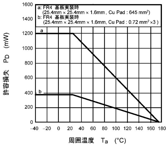
図 8.11 P_D - T_a
