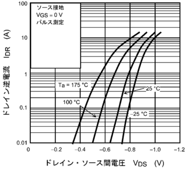
図 9.7 I_{DR} - V_{DS}
