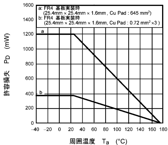
図 9.13 P_D - T_a
