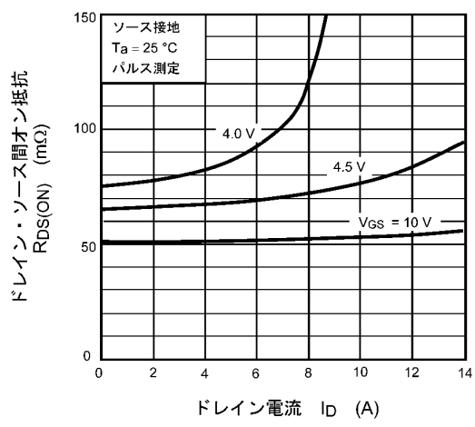
図 7.4 R_{DS(ON)} - I_D
