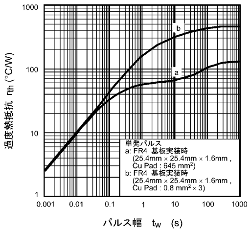
図 7.12 rth - tw
