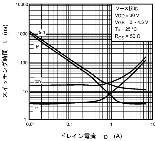
図 8.9 t - I_D
