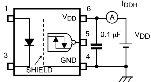
図 12.1.4 IDD_H測定回路
