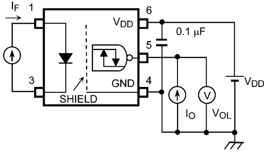
図 12.1.1 VOL測定回路
