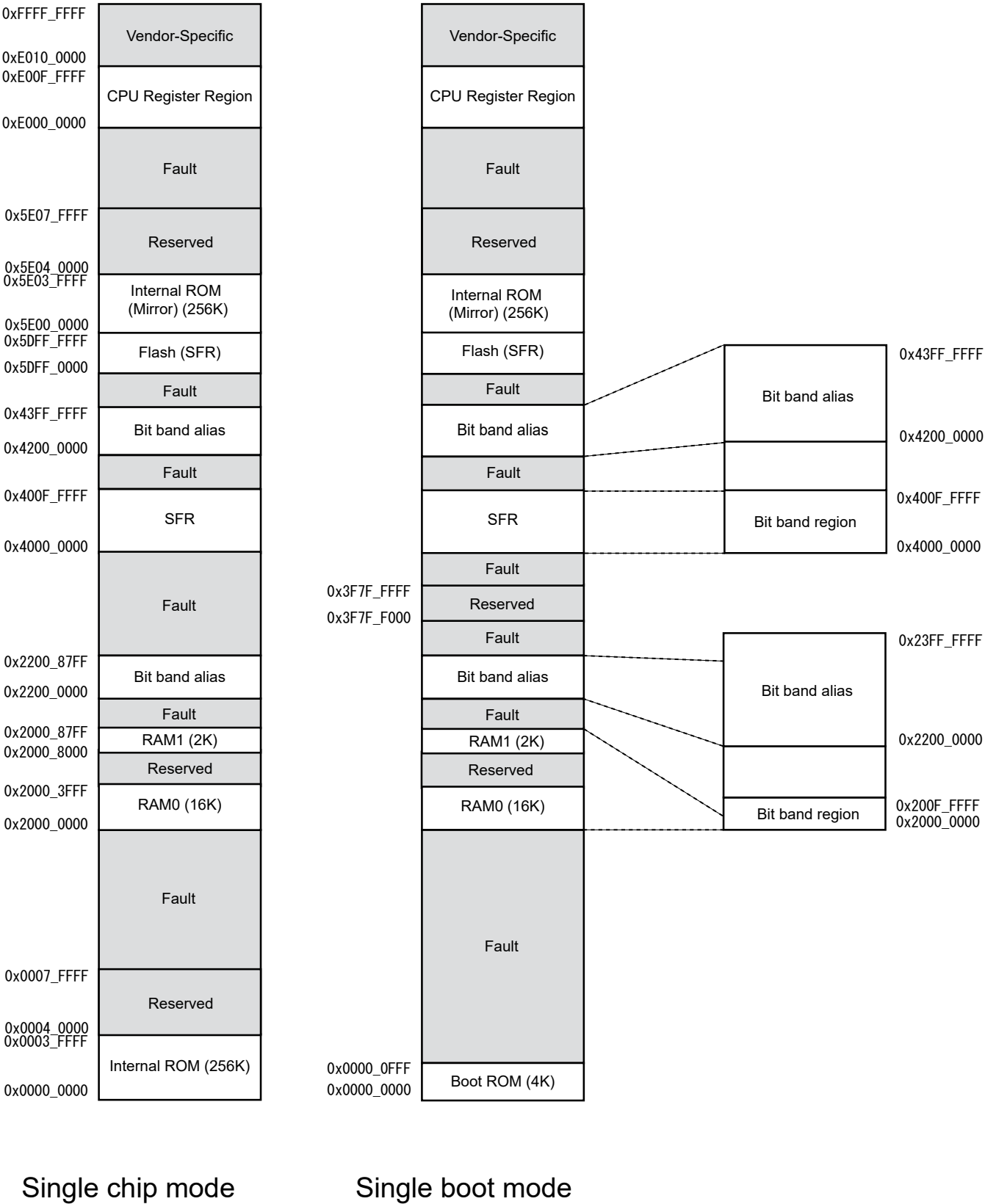
Figure 4-3 MemoryMap(256KB)
