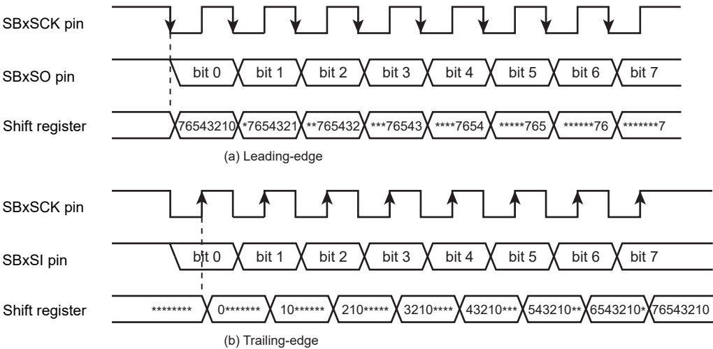
Figure 14-15 Shift Edge
