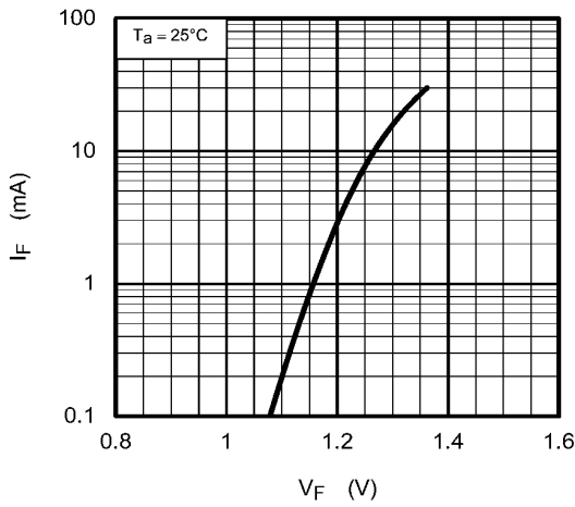
図 14.1.3 I_F - V_F
