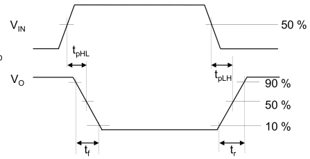
図 12.1.5 伝搬遅延時間測定回路, 波形
