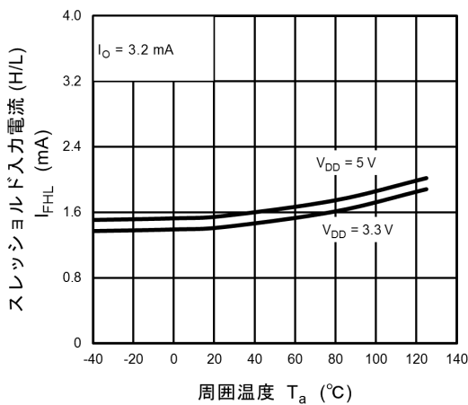
図 12.2.9 I_{FHL} - T_a
