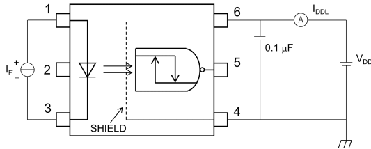
図 12.1.3 I DDL 測定回路
