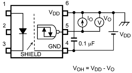
図 12.1.2 VOH測定回路
