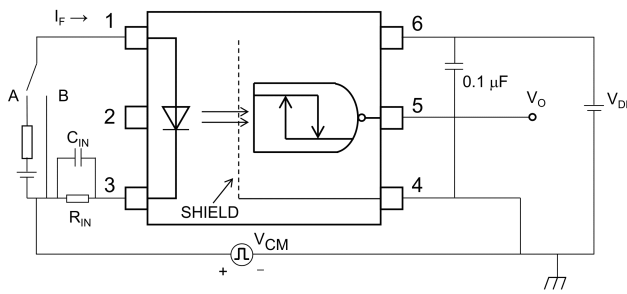
図 12.1.6 コモンモードノイズ除去電圧測定回路, 波形
