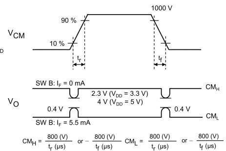
図 12.1.6 コモンモードノイズ除去電圧測定回路, 波形
