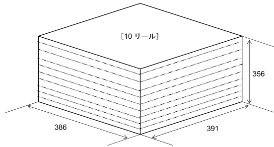
10リール入り梱包箱 (unit: mm)
