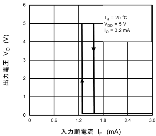
図 12.2.11 V_O - I_F
