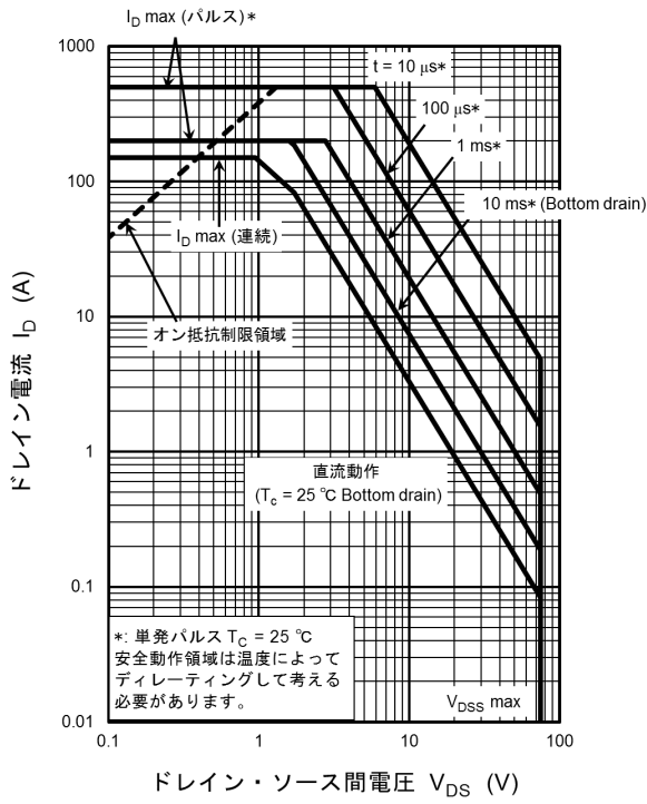
図 8.16 安全動作領域 (最大値 (保証値))
