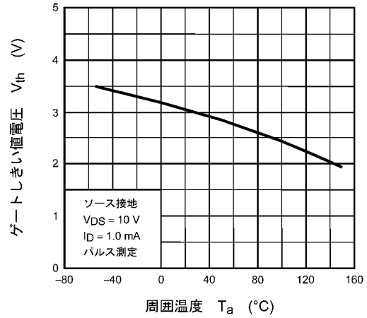
図 8.8 V_{th} - T_a
