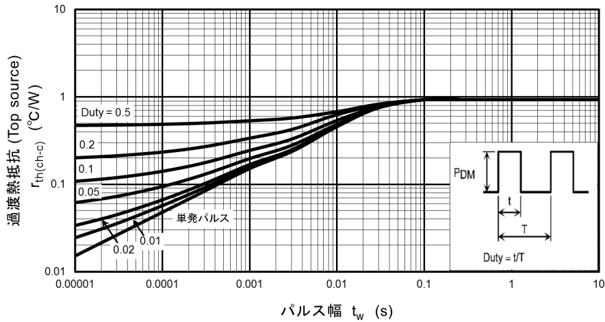
図 8.13 r_{th} - t_w (Top source) (最大値 (保証値))
