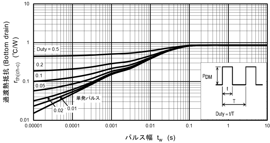
図 8.12 r_{th} - t_w (Bottom drain) (最大値 (保証値))
