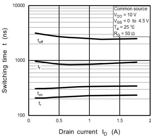
Fig. 7.9 t - I_D
