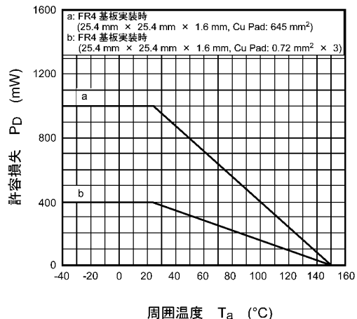
図 7.12 P_D - T_a
