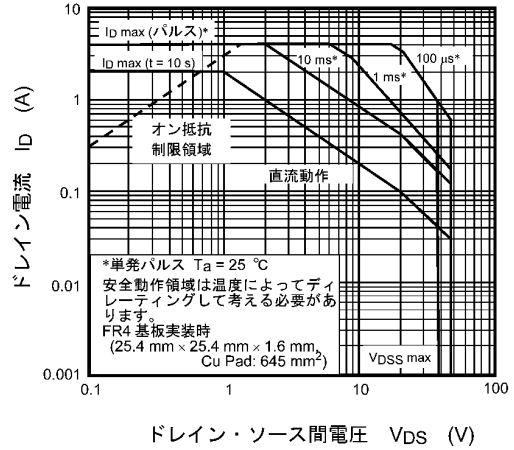
図 7.10 安全動作領域
