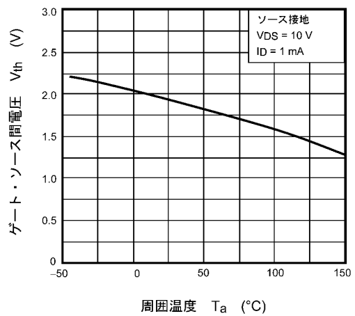
図 7.6 V_{th} - T_a
