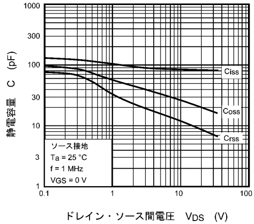
図 7.8 C - V_{DS}
