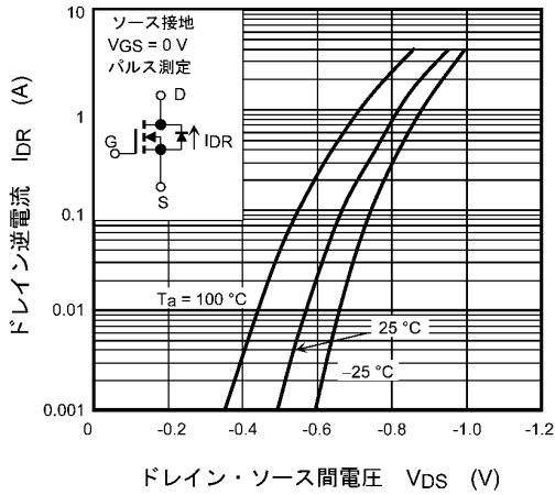
図 7.7 I_{DR} - V_{DS}
