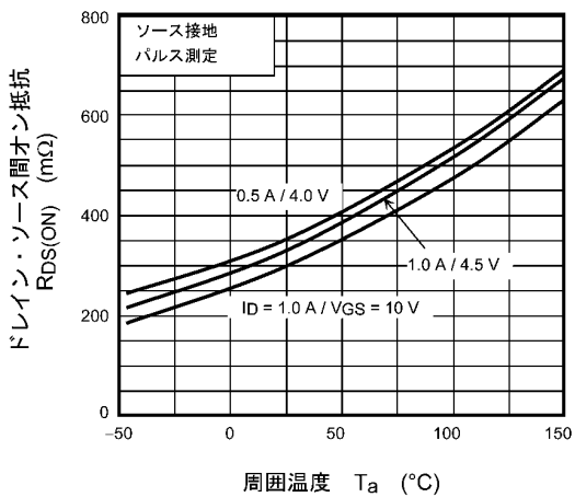
図 7.5 R_{DS(ON)} - T_a
