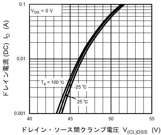
図 7.13 I_D - V_{(CL)DSS}
