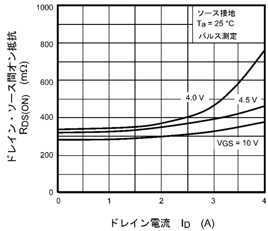
図 7.4 R_{DS(ON)} - I_D
