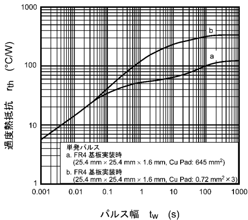
図 7.11 r_{th} - t_w
