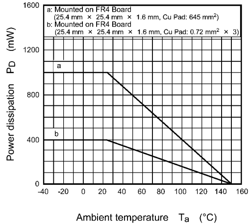
Fig. 7.12 PD - Ta
