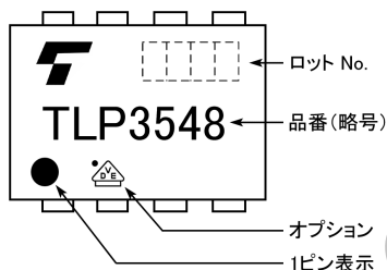
図 20.3 オプションマーク入り現品表示 (VDE認定品) (注)
