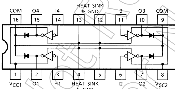
TD62308BFG
