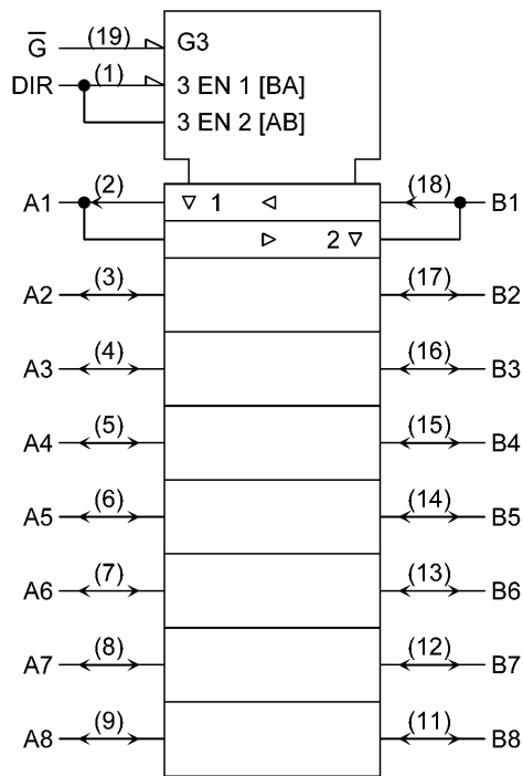
TC74ACT245P
