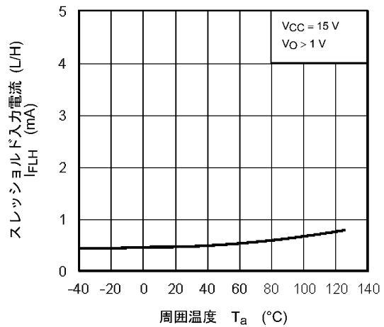
図 12.2.4 I_{FLH} - T_a
