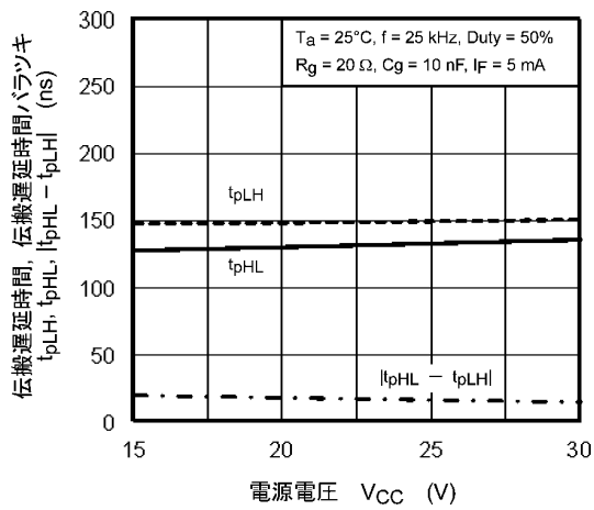
図 12.2.15 t_{PLH} , t_{PHL} , |t_{PHL} - t_{PLH}| - V_{CC}
