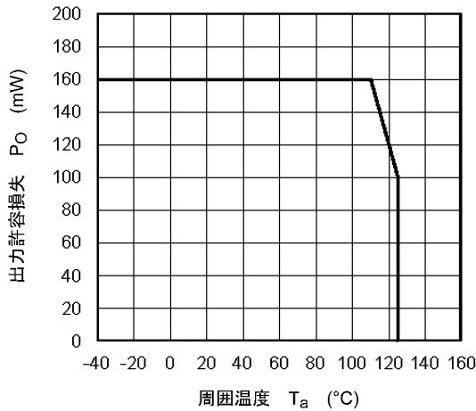
図 12.2.3 P_O - T_a
