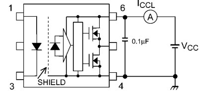
図 12.1.6 ICCL測定回路
