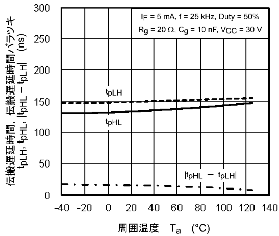
図 12.2.13 t_{PLH} , t_{PHL} , |t_{PHL} - t_{PLH}| - T_a
