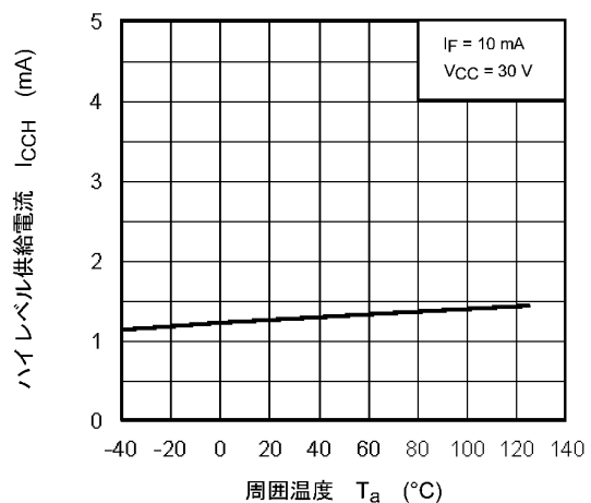
図 12.2.6 I_{CCH} - T_a
