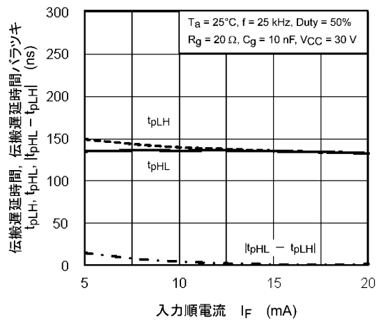
図 12.2.14 t_{PLH} , t_{PHL} , |t_{PHL} - t_{PLH}| - I_F
