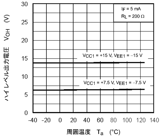
図 12.2.8 VOH - Ta
