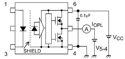
図 12.1.2 IOPL測定回路
