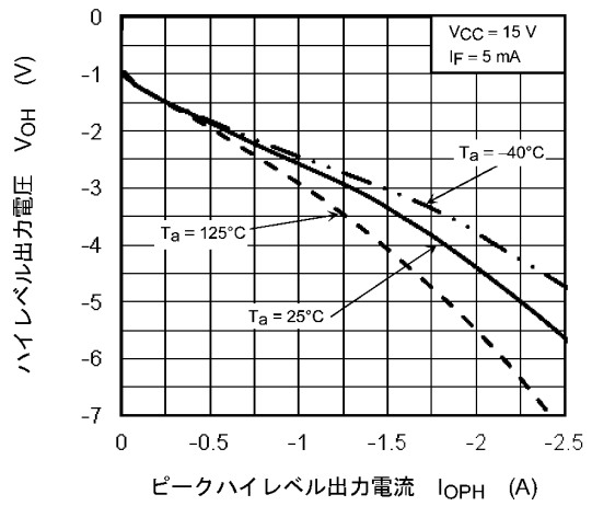
図 12.2.10 VOH - IOPH
