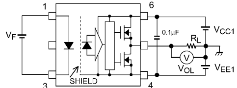
図 12.1.4 VOL測定回路
