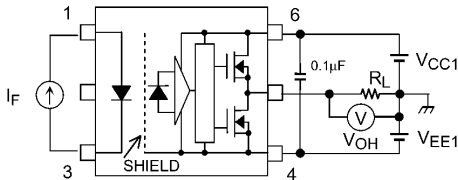
図 12.1.3 VOH測定回路
