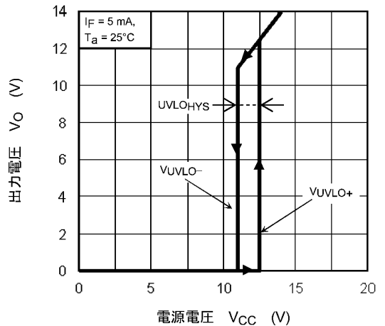
図 12.2.12 VO(VUVLO) - VCC
