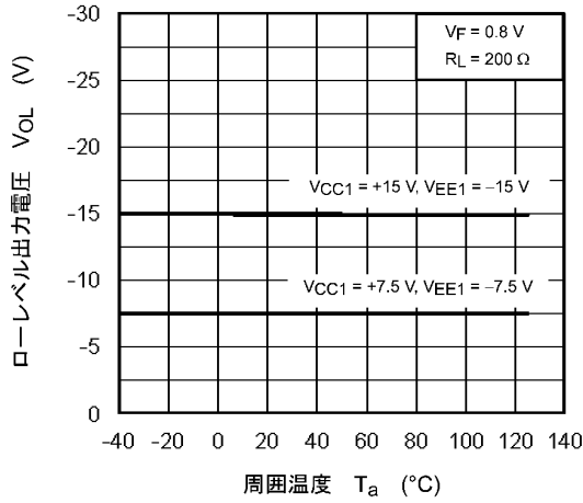
図 12.2.7 VOL - Ta
