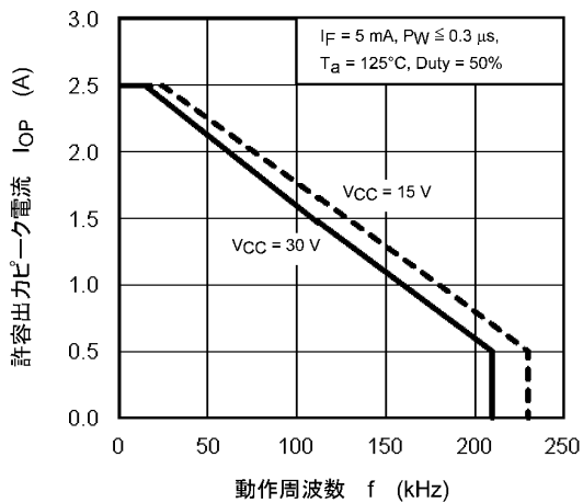
図 12.2.11 IOP - f
