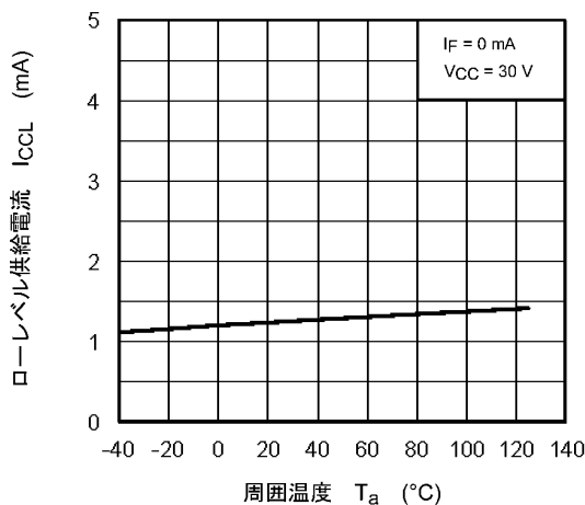
図 12.2.5 I_{CCL} - T_a
