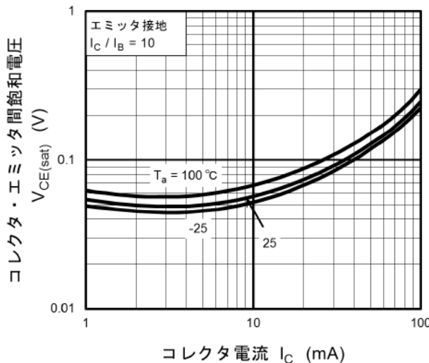
図 11.23 RN1105MFV V_{CE(sat)}-I_C
