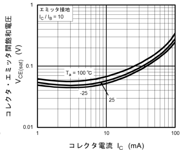
図 11.24 RN1106MFV V_{CE(sat)}-I_C
