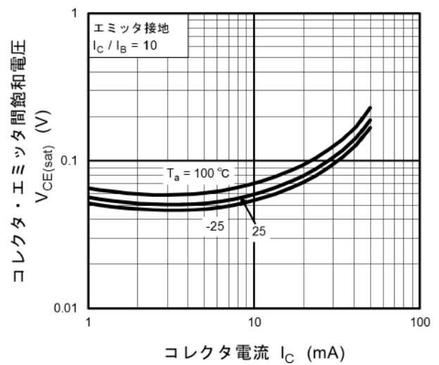
図 11.22 RN1104MFV V_{CE(sat)}-I_C
