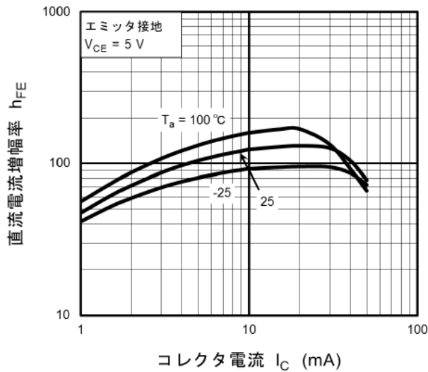
図 11.7 RN1107MFV h_{FE} - I_C
