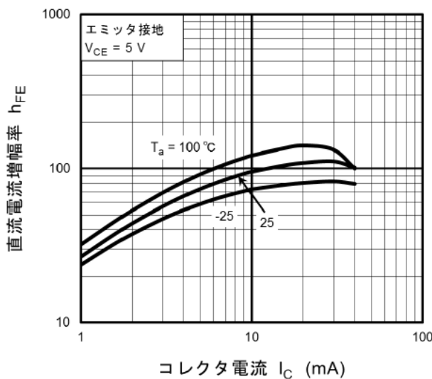
図 11.9 RN1109MFV h_{FE} - I_C
