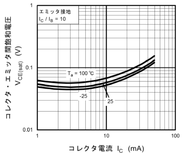
図 11.12 RN1109MFV V_{CE(sat)} - I_C
