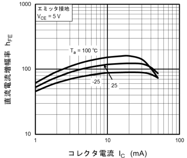
図 11.8 RN1108MFV h_{FE} - I_C
