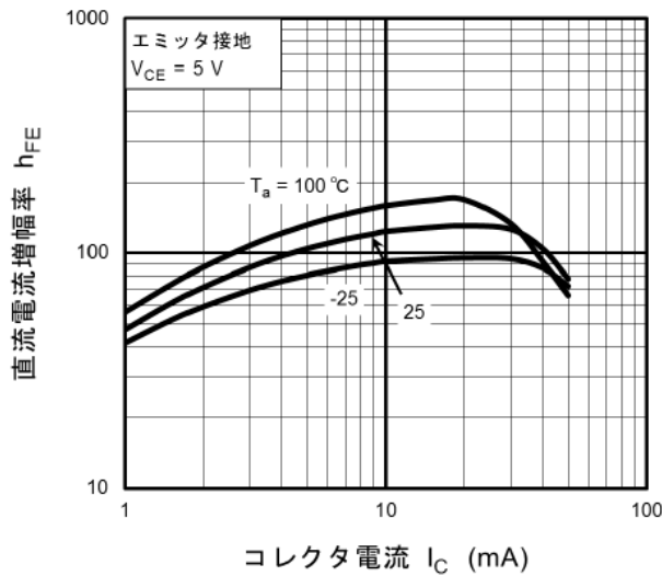
図 11.7 RN1107MFV h_{FE} - I_C
