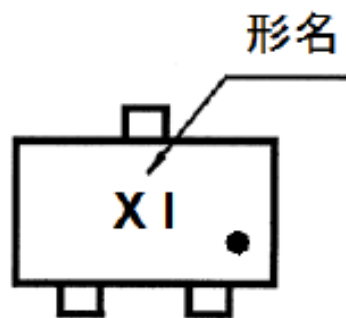
图 10.2 現品表示 RN1108MFV
