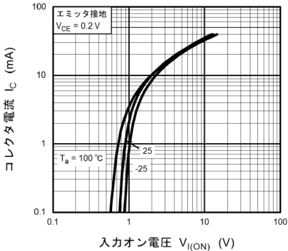
図 11.1 RN1107MFV I_C - V_{I(ON)}
