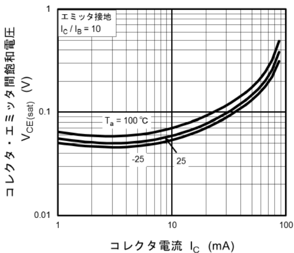
図 11.11 RN1108MFV V_{CE(sat)} - I_C
