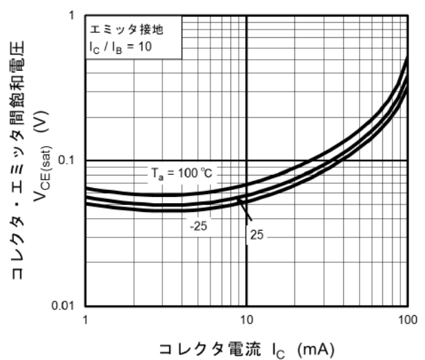
図 11.10 RN1107MFV V_{CE(sat)} - I_C
