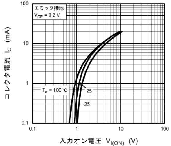
図 11.2 RN1108MFV I_C - V_{I(ON)}
