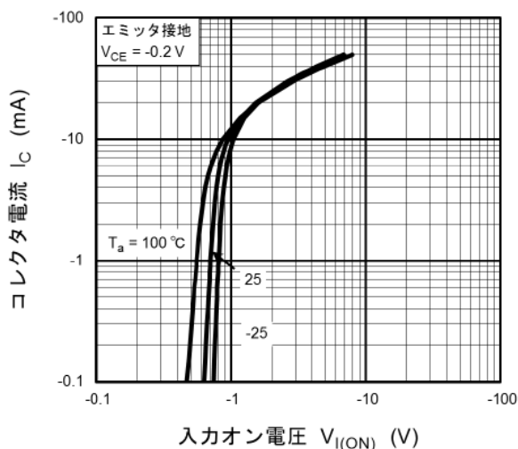
図 11.5 RN2105MFV I_C - V_{I(ON)}
