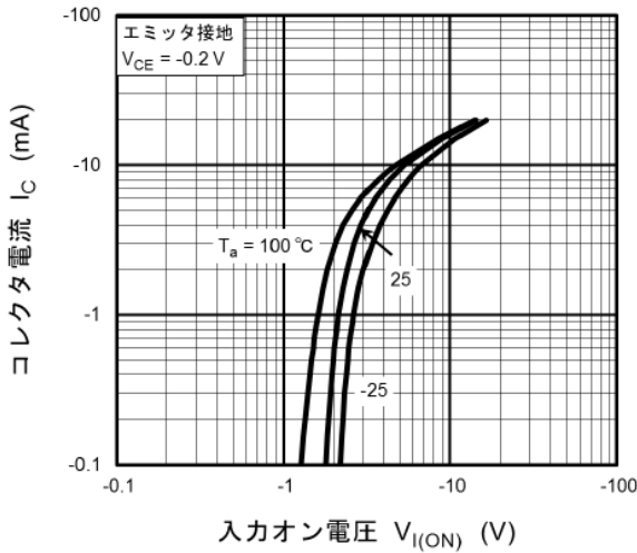
図 11.1 RN2107MFV I_C - V_{I(ON)}
