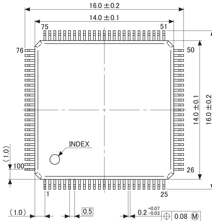
外形寸法図
