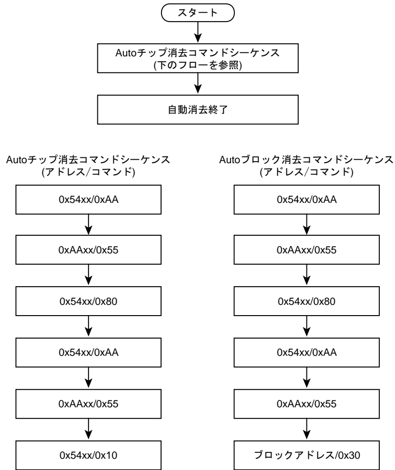
図 17-13 自動消去
