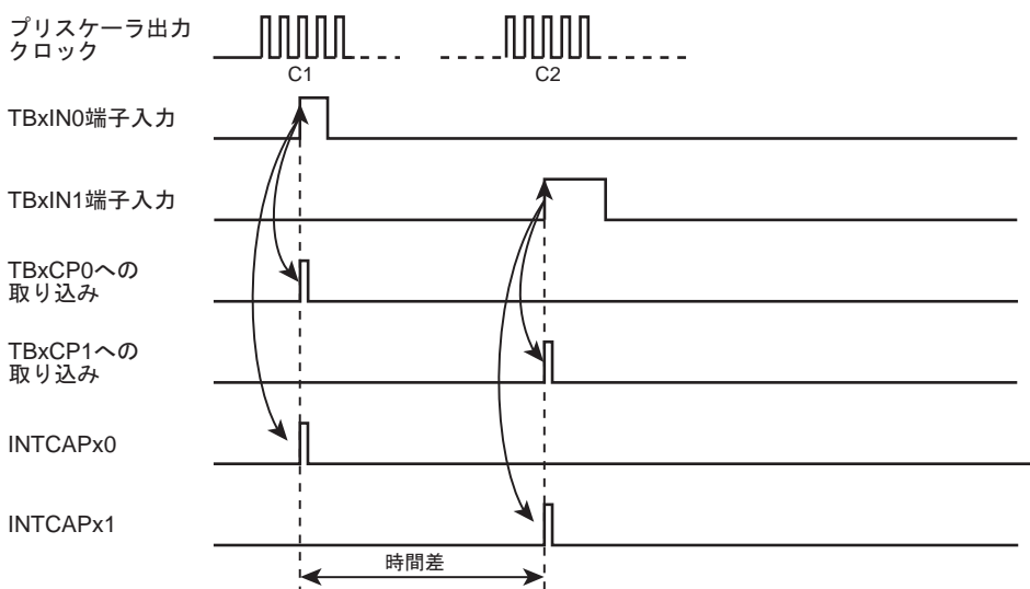
図 9-9 時間差測定
